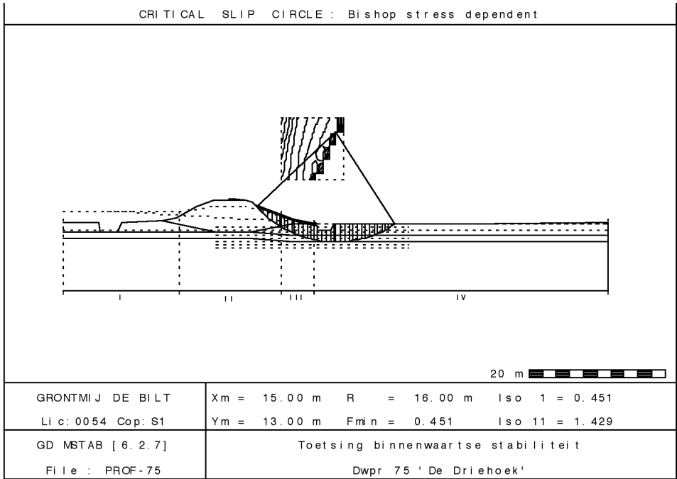
Figuur A 6 Toetsing macrostabiliteit binnenwaarts
