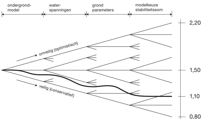
Figuur 10 Schematiseringstrein stabiliteitsanalyse dijken
