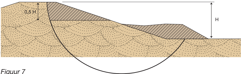
Figuur 7 Veronderstelde eindsituatie na afschuiving langs primair glijvlak
