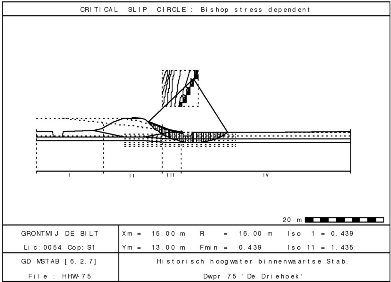
Figuur A 8 Veiligheidsfactor voor HHW-omstandigheden, met karakteristieke sterktewaarden
