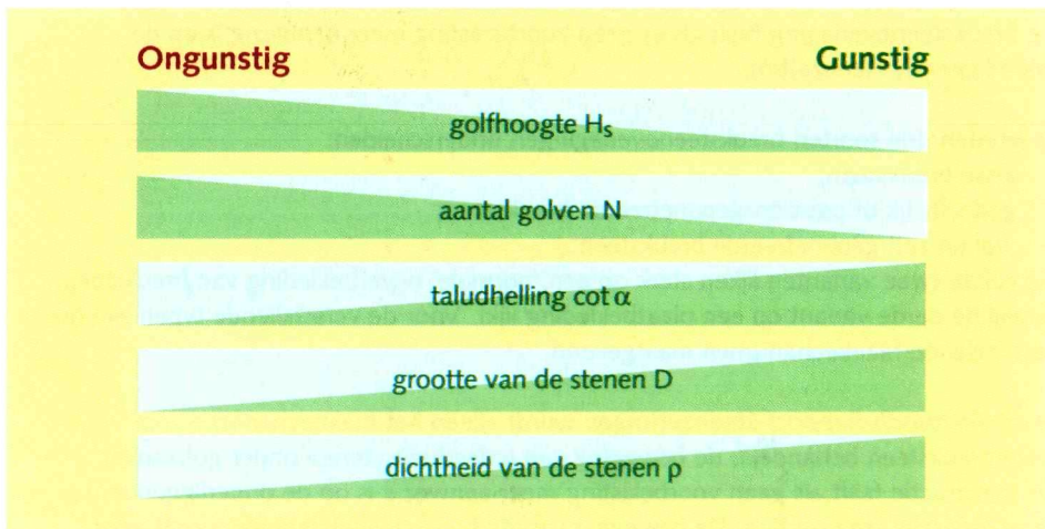
Figuur 3.16 Parameters breuksteenoverlaging
