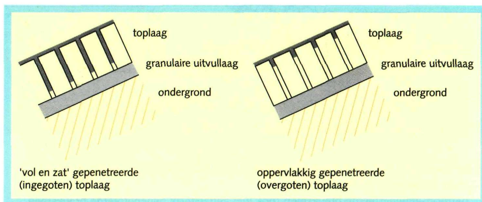
Figuur 2.4 Definities gepermeerde toplaag
