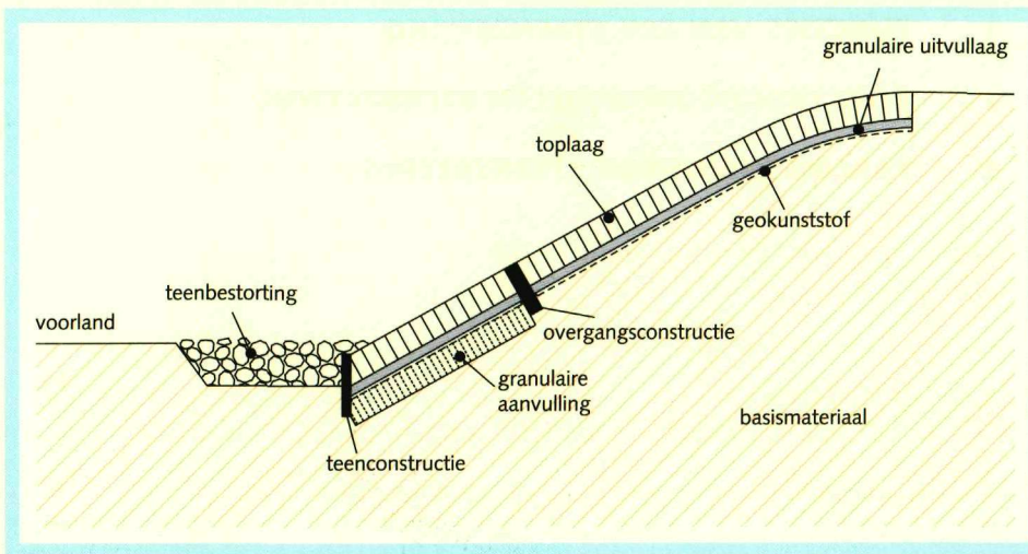
Figuur 1.1 Opbouw van een bekledings- systeem
