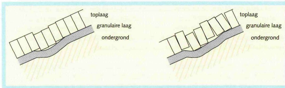
Figuur 3.11 Schadeverloop bij faalmechanisme materiaaltransport vanuit de ondergrond
