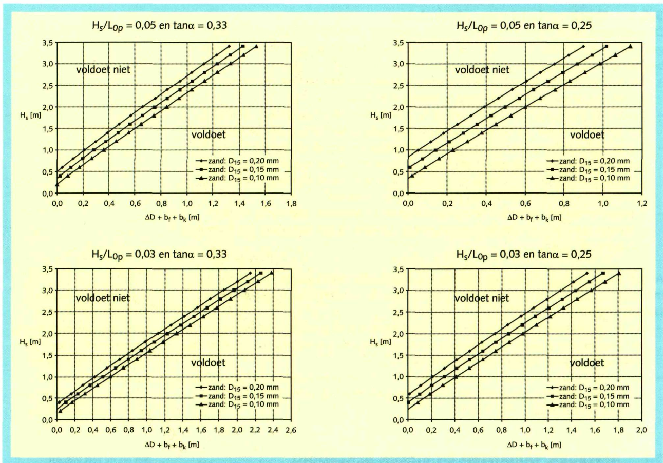
Figuur 5.4 Rekenregel voor de weerstand tegen afschuiving
