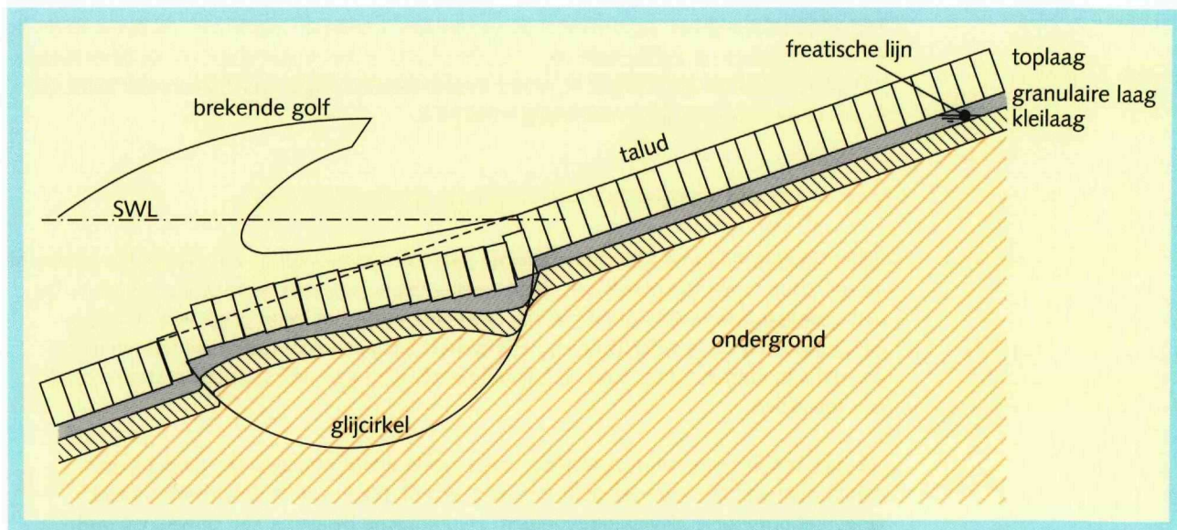
Figuur 3.8 Diepe kleinschalige afschuiving
