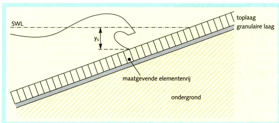
Figuur B.1 Bepaling maatgevende waterstand
