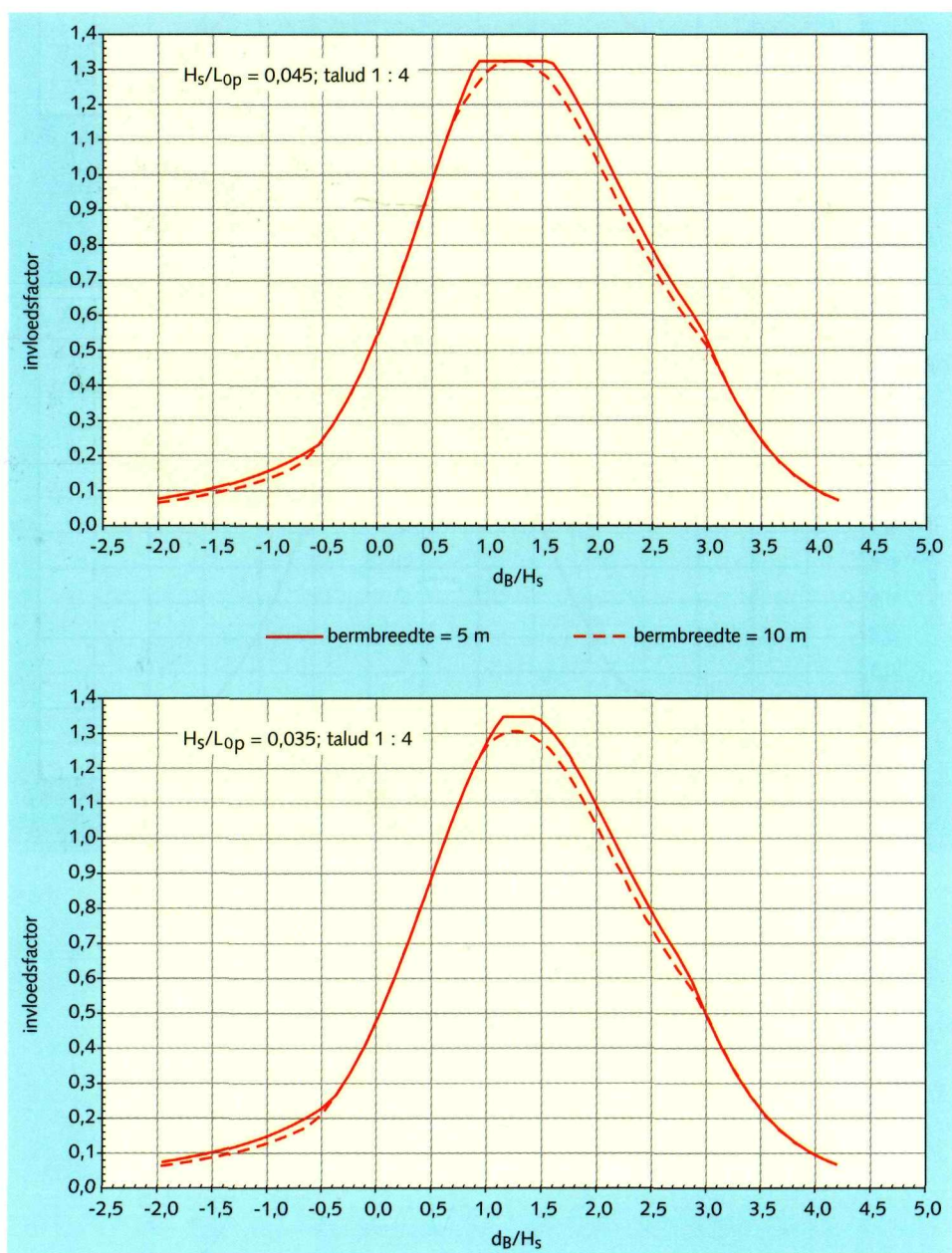
Figuur H.2 Bermfactor voor taludhelling onder de berm 1:4
