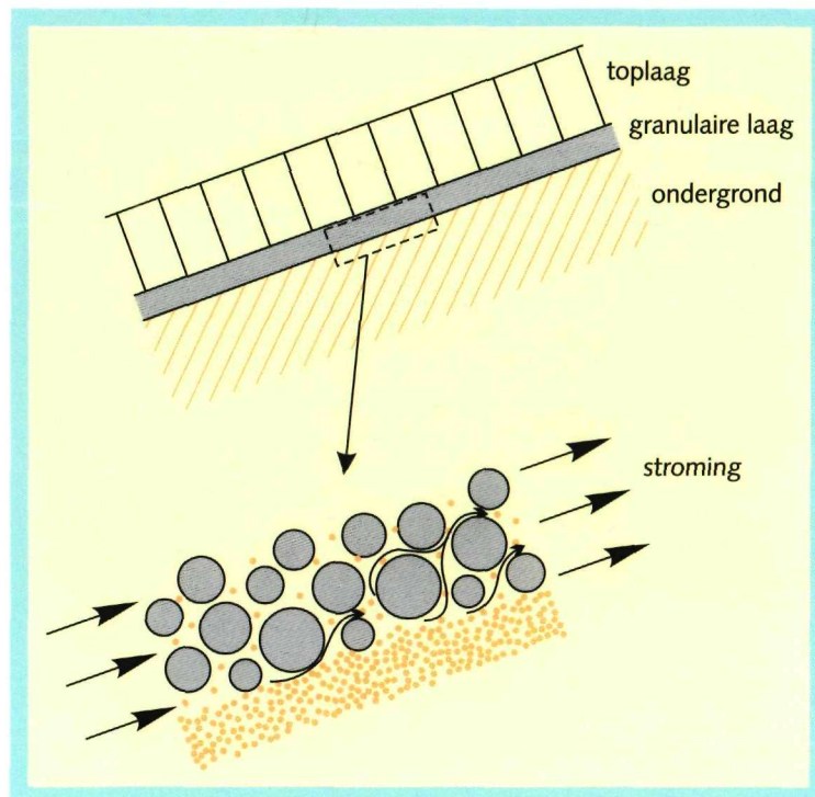
Figuur 3.10 Uitspoeling van materiaal uit de onderlaag
