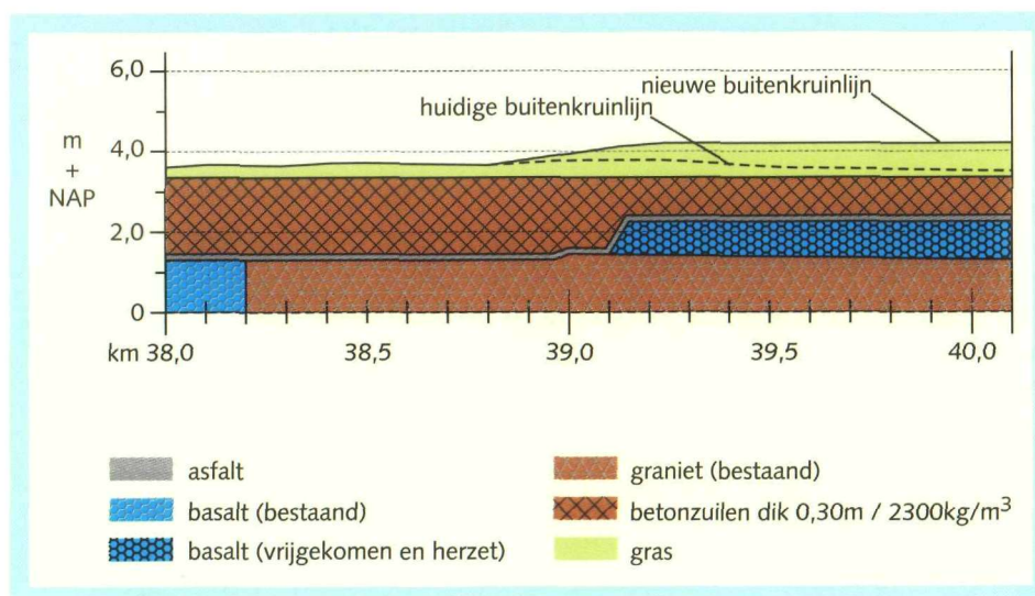
Figuur 9.2 Glooiingskaart Ramsdijk
