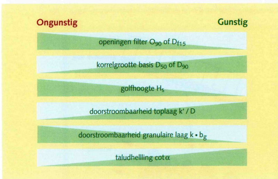
Figuur 3.12 Parameters materiaaltransport ondergrond > granulaire laag
