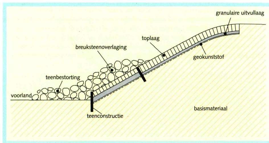
Figuur 2.5 Overlaging met losse breksteen
