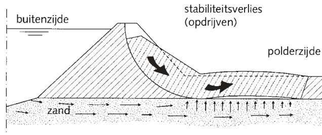
Figuur 5.3.3 Opdriven
