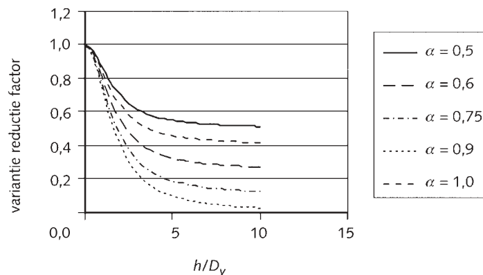
Figuur 1.3.2 Variantiereductiefactor voor uitmiddeling in verticale richting
