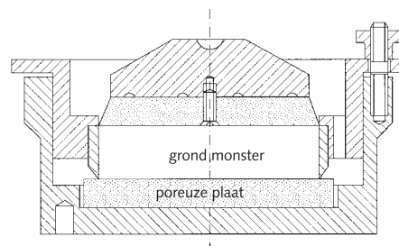
Fig. 6.1 Samendrukkingsproef
