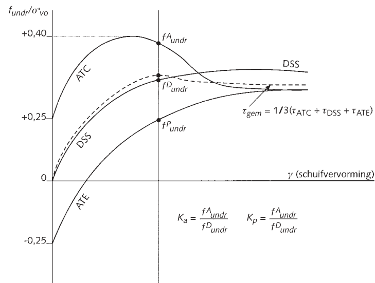
Figuur 2.4 Bepaling ongedraineerde schuifsterkte ( f_{undr}^A , f_{undr}^D en f_{undr}^P ), rekening houdend met de compabiliteit van de rek en uitgaande van een star glijvlak
