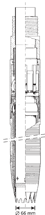
Figuur 3.2 Continuu-steekapparaat
