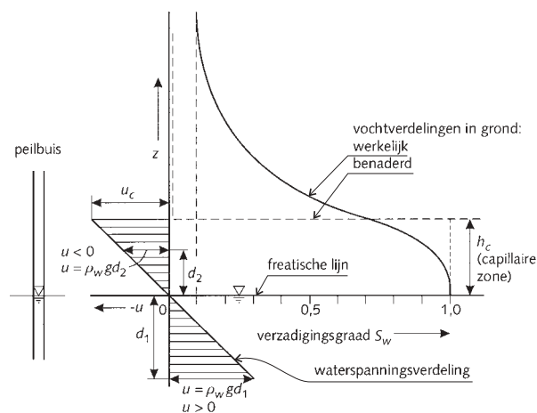
Figuur 4.5.3 Capillaire zone
