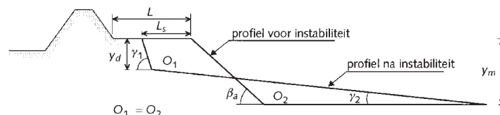
Figuur 5.7.1 Twee-dimensionaal bergingsmodel met onbeperkte berging
