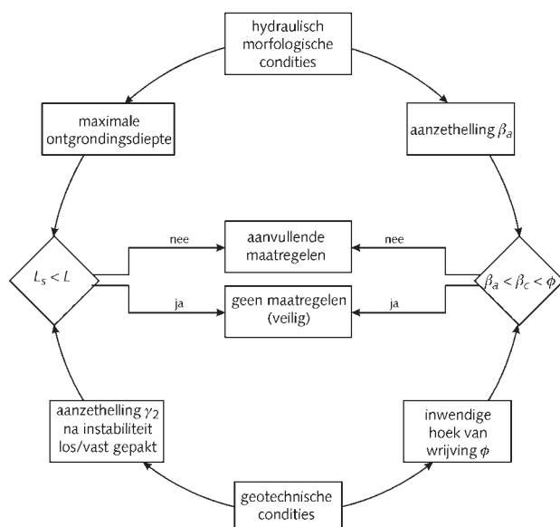
Figuur 5.7.2 Relatie tussen sterkte en belastingparameters
