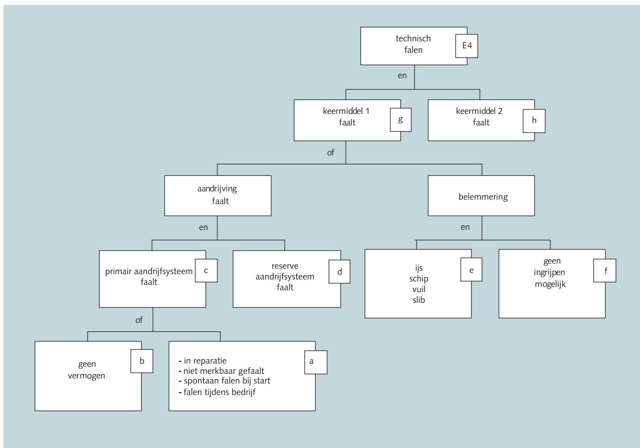
Figuur B3.12 Uitwerking tak 'technisch falen'
