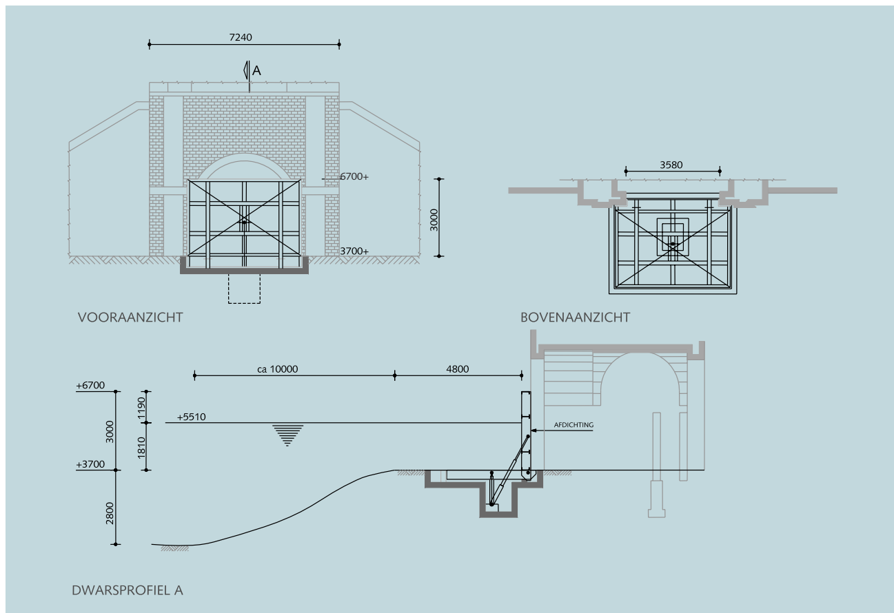
Figuur B5.8 Coupure
