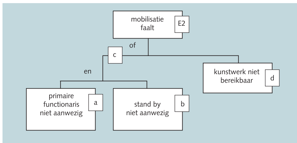
Figuur B3.10 Uitwerking tak 'mobilisatie faalt'
