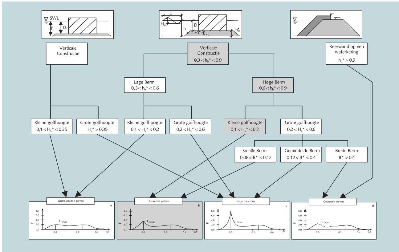
Figuur B5.9 Keuze belastingmodel voorbeeld coupeure
