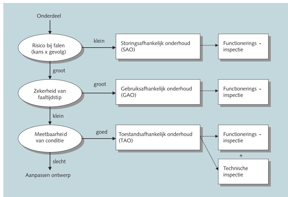
Figuur B6.6 Beslisdigram onderhouds- en inspectiestrategie
