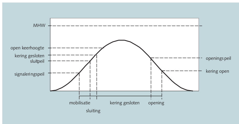
Figuur B3.3 Waterstandsverlooplijn en belangrijkste peilen
