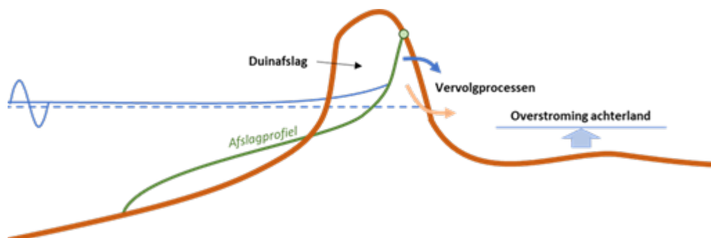
Figuur 1 Schematische weergave van het initieel mechanisme (duinafslag) en eventuele vervolgemechanismen (golfoploop/overslag en geotechnische instabiliteit) van het faalpad duinafslag.
