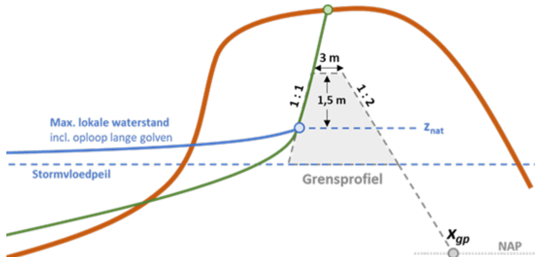
Figuur 1 Schematische weergave van de vorm en de dimensies van het grensprofiel.
