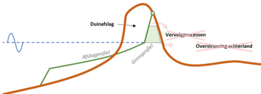
Figuur 2 Voorbeeld van de rol van het grensprofiel in een duinwaterkering: het grensprofiel is het minimaal benodigde resterende profiel ná duinafslag om te voorkomen dat vervolgprocessen kunnen resulteren in een doorbraak van de zandige waterkering en overstroming van het achterland.
