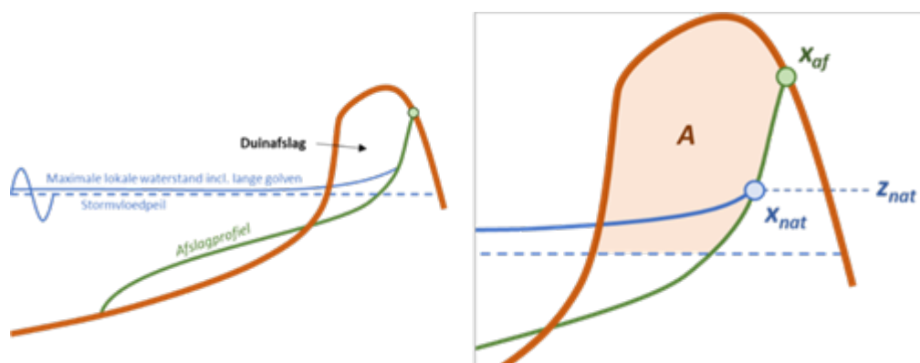
Figuur 1 Schematische weergave van enkele relevante uitvoerparameters van het XBeach-BOI-model: het afslagprofiel (groen), het afslagvolume ( A ), het afslagpunt ( x_{af} ) en het maatgevende olopunt ( x_{nat}, z_{nat} ).
