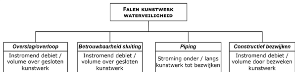
Figuur 1 Vigerende faalboom kunstwerken waterveiligheid.
