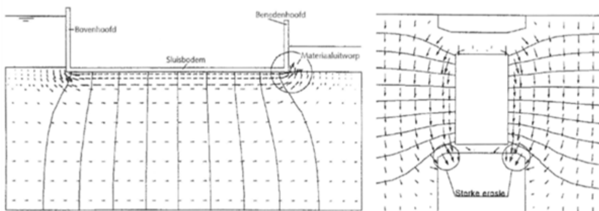
Figuur 1 Links: onderloopsheid bij een kunstwerk (schematisatie langsdoorsnede). Rechts: achterloopsheid bij een kunstwerk (schematisatie bovenaanzicht). Beide figuren zijn ontleend aan
