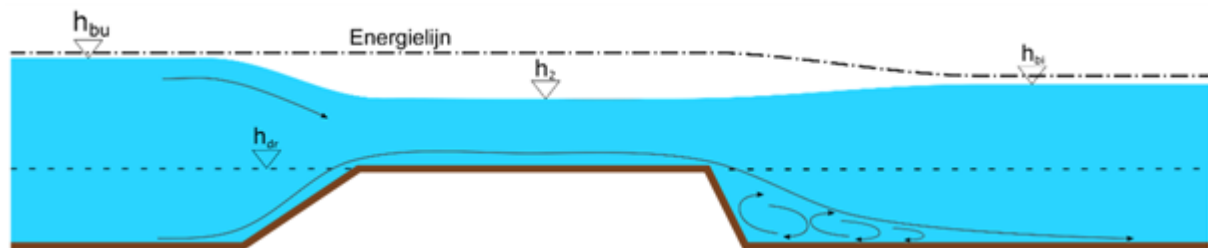
Figuur 1 Onvolkomen overlaat.
