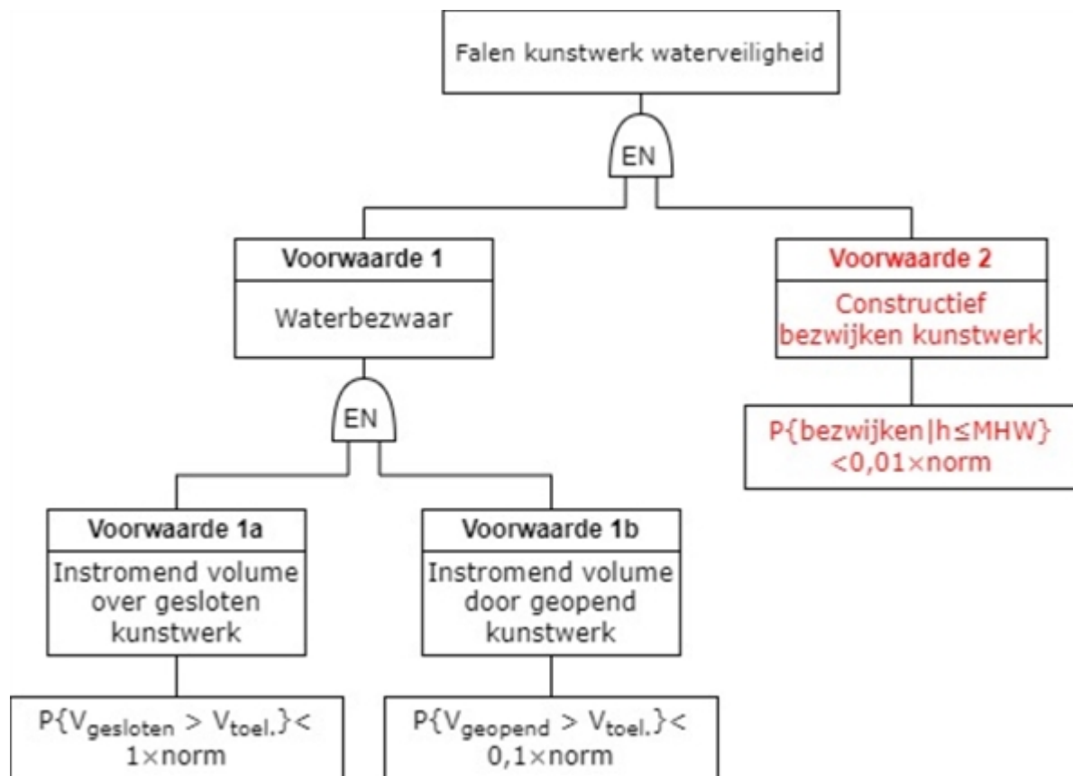
Figuur 1 Faalpaden op hoofdlijnen volgens Leidraad kunstwerken 2003. In het rood het pad voor piping. [3]
