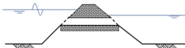
Figuur 1 Schematische weergave van de diverse instromingsmodellen bij betrouwbaarheid sluiting.
