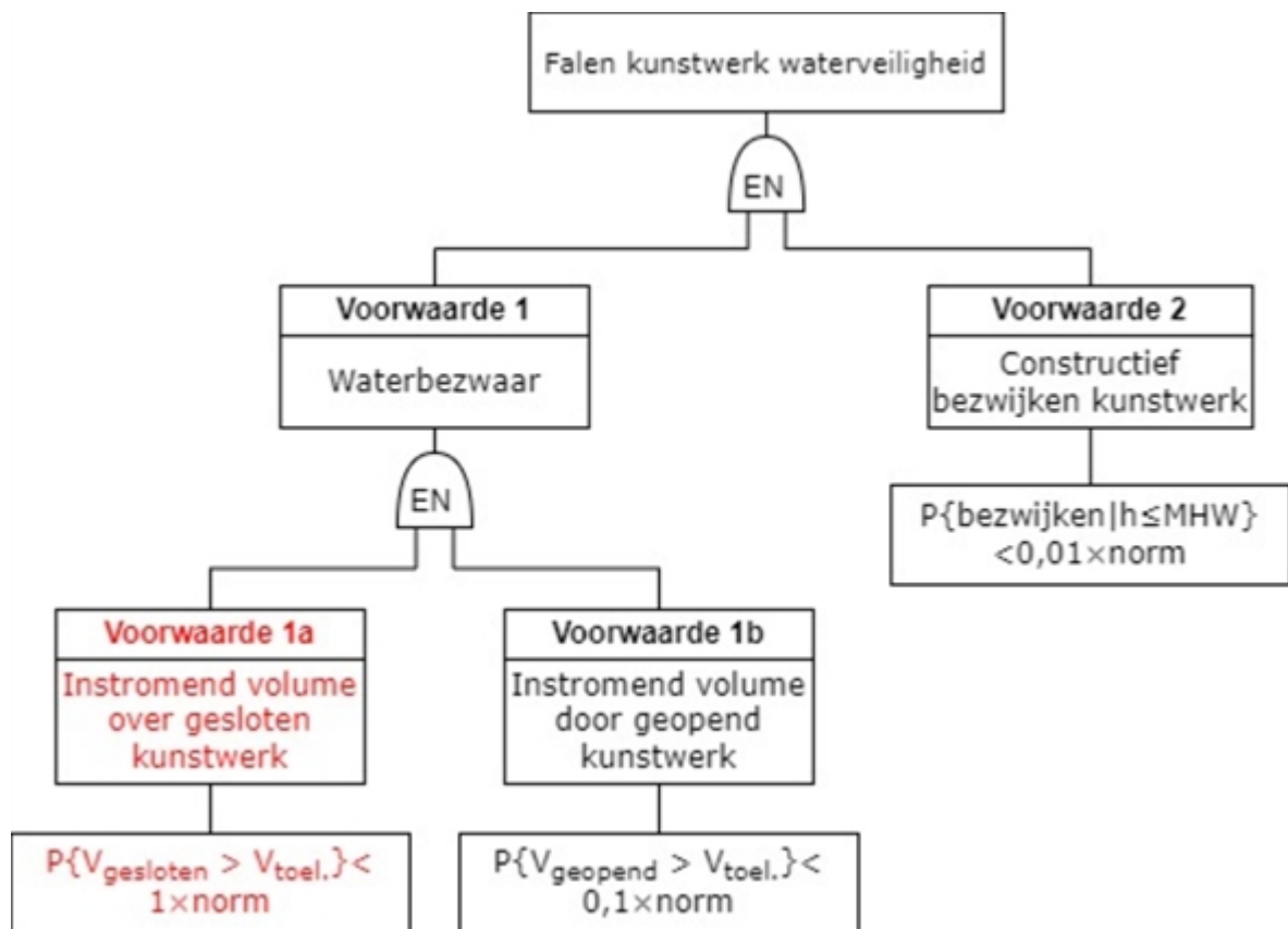
Figuur 1 Faalpaden op hoofdlijnen volgens Leidraad kunstwerken. Voorwaarde 2 is van toepassing op sterkte en/of stabiliteit.
