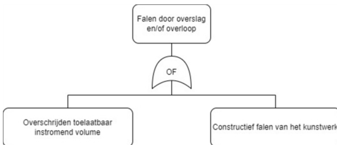
Figuur 2 Falen door overslag en/of overloop conform Leidraad kunstwerken.
