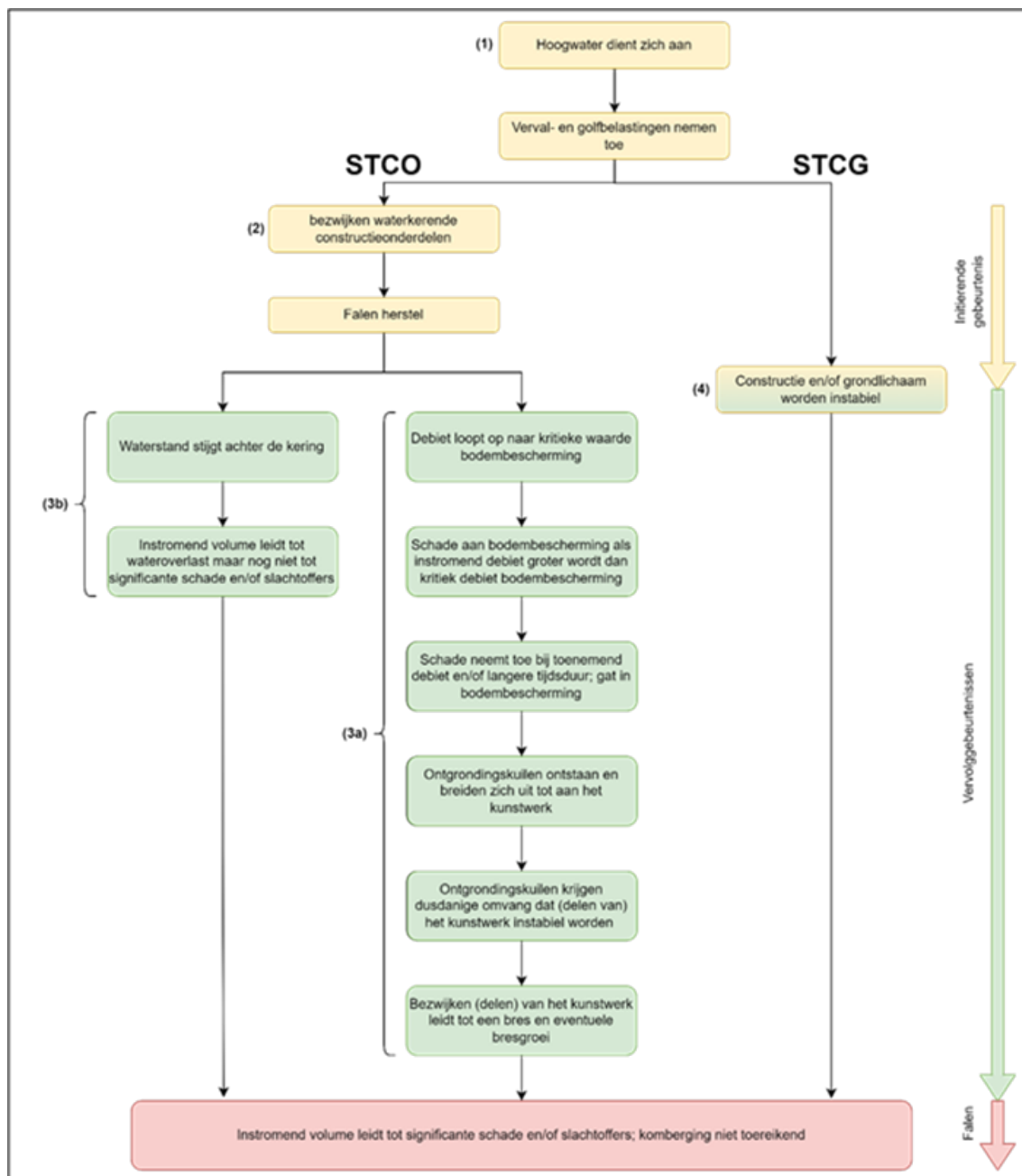
Figuur 1 Faalproces Sterkte en/of Stabiliteit
