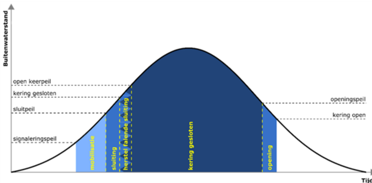
Figuur 1 Schematisch verloop sluitingsproces bij een hoogwatergolf (uitgangspunt is dat het kunstwerk niet hoogwaterkerend gesloten is op het moment dat de hoogwatergolf aankomt). In de figuur is de buitenwaterstand waarbij ongewenste instroming plaatsvindt aangeduid als 'open keerpeil'.
