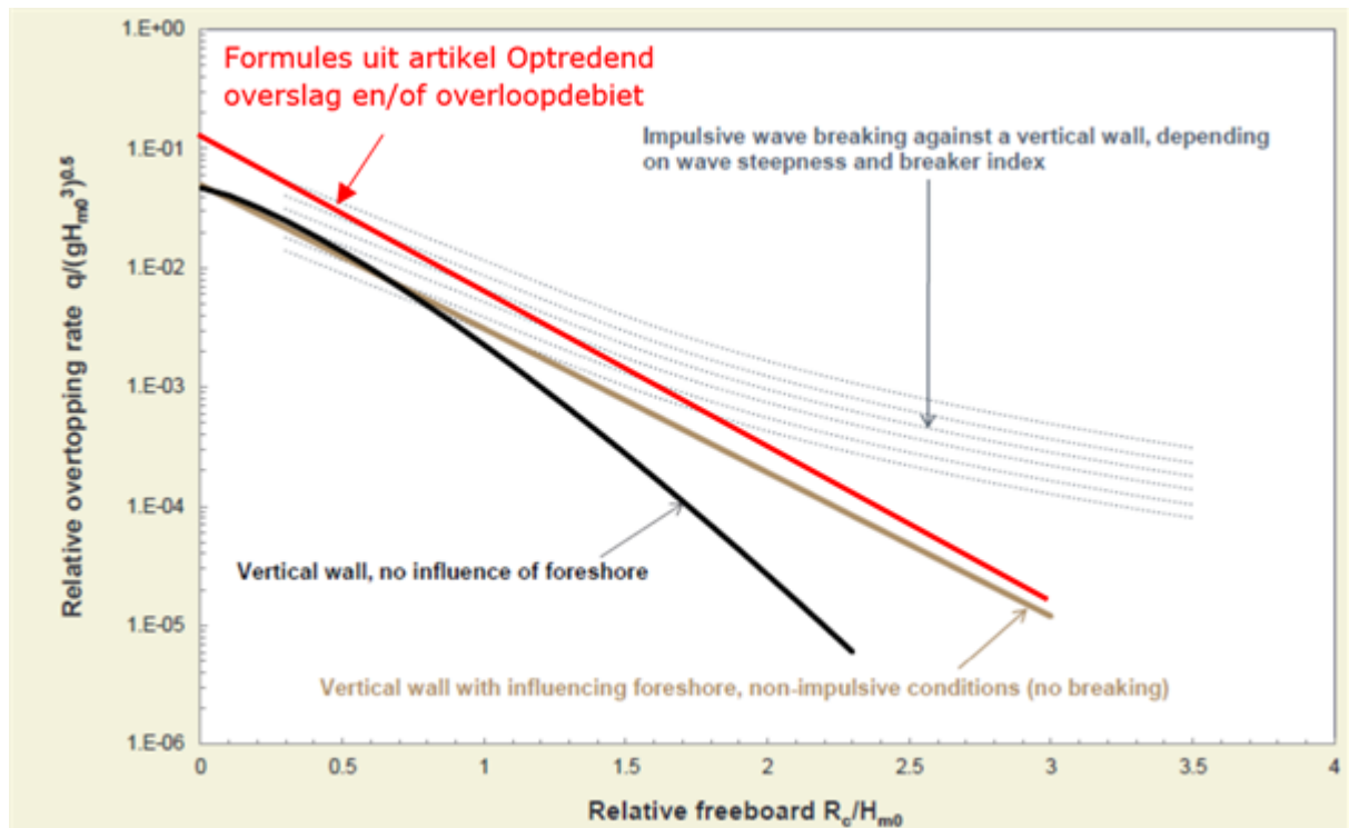
Figuur 1 Overzicht formules in grafische vorm voor verticale constructies uit EurOtop 2018 en artikel Optredend overslag- en/of overloopdebiet. Het vrijboord ( R_c ) is de hoogte van de kruin boven de lokale stilwaterstand. Basis: figuur 7.5 uit EurOtop 2018, de rode lijn is hieraan toegevoegd.
