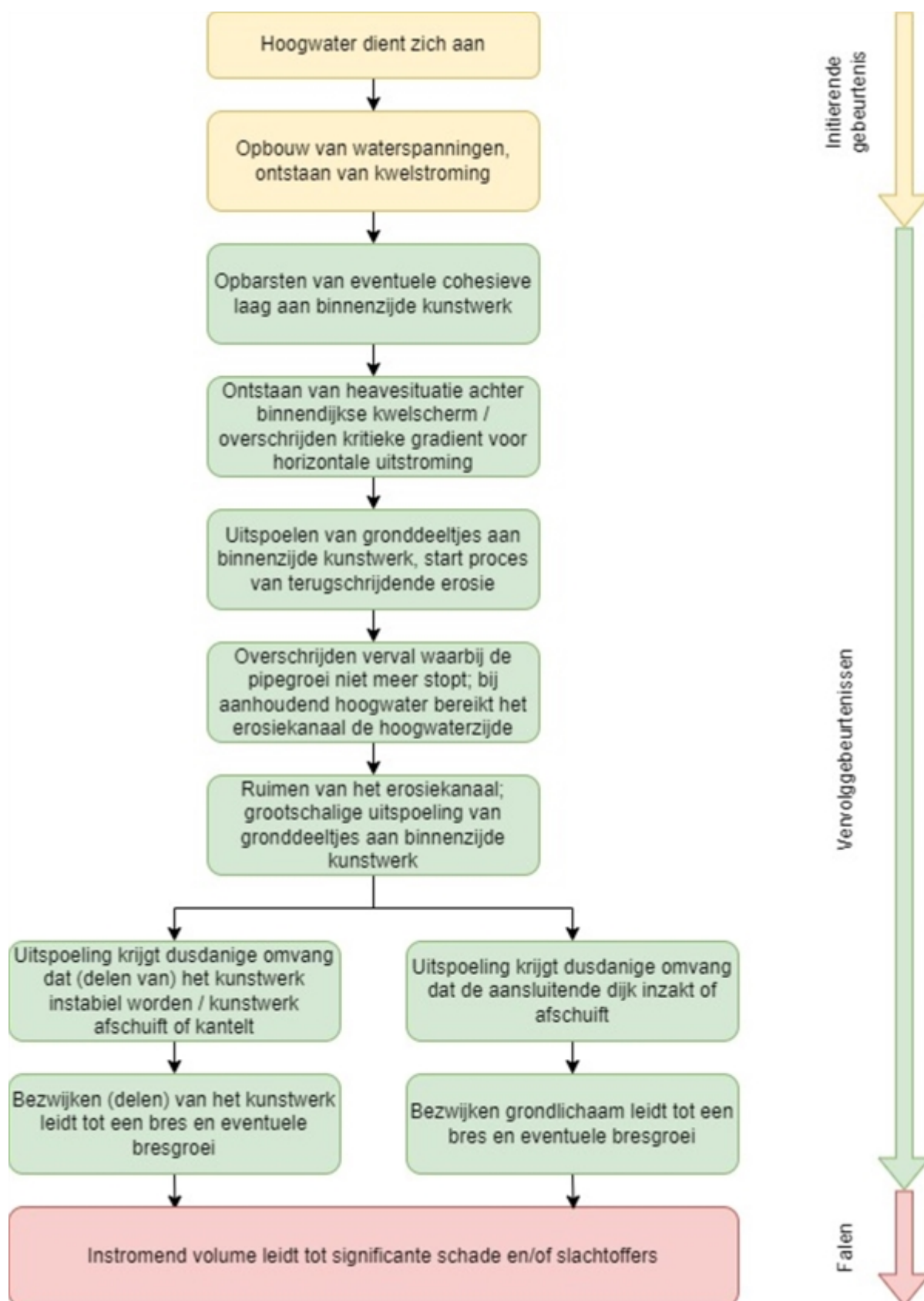
Figuur 1 Faalproces piping bij kunstwerk.
