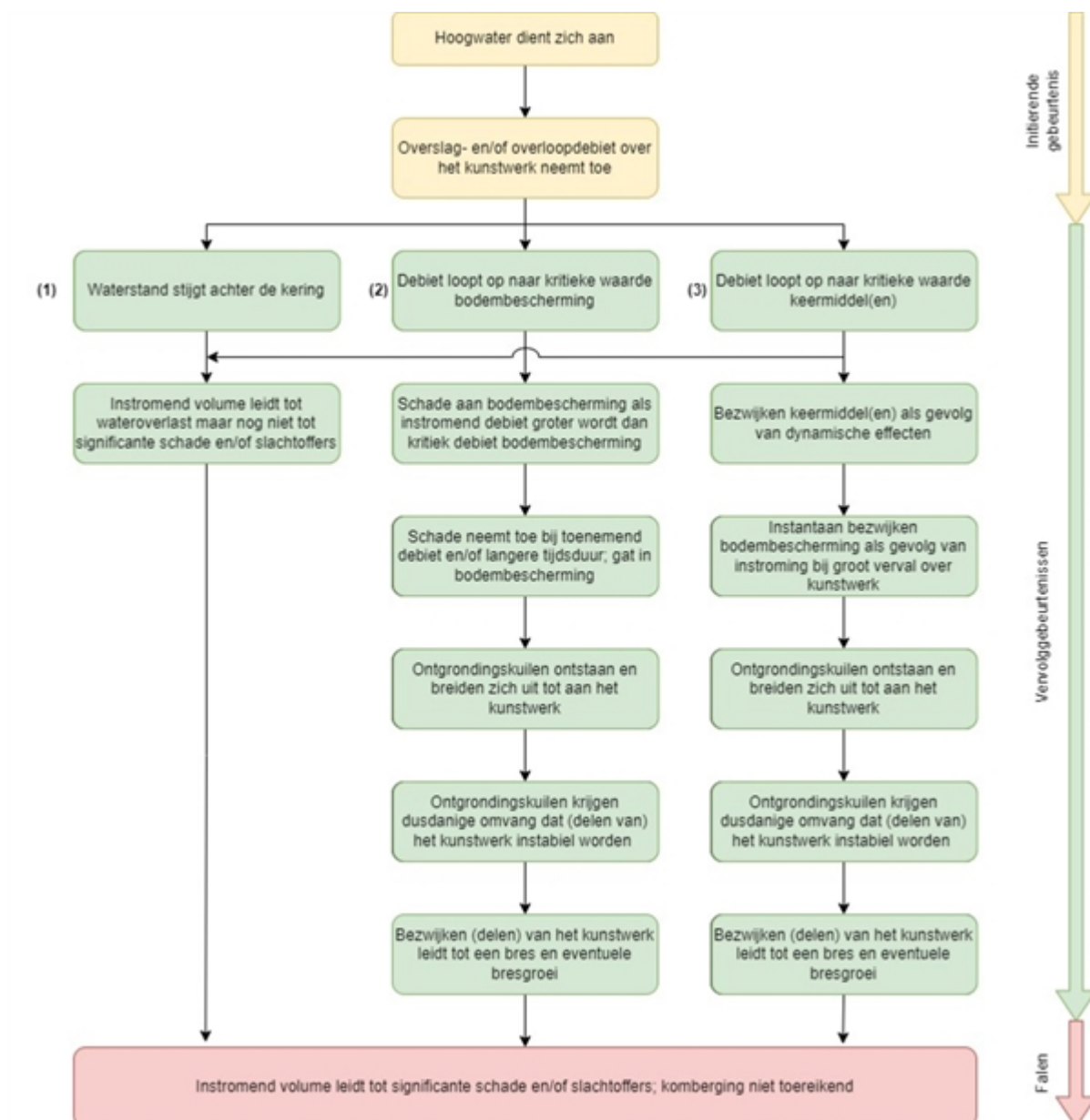
Figuur 1 Faalproces overslag en/of overloop.
