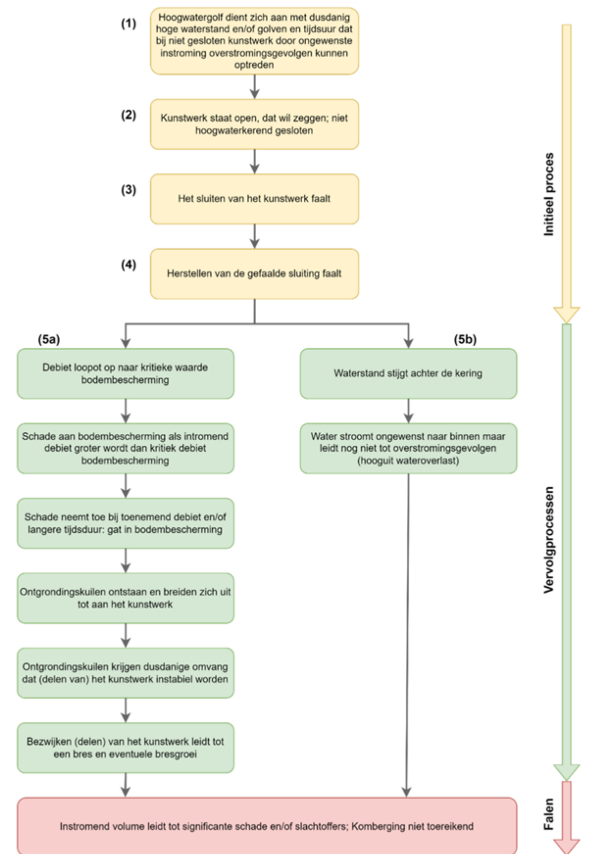
Figuur 1 Faalproces betrouwbaarheid sluiting.
