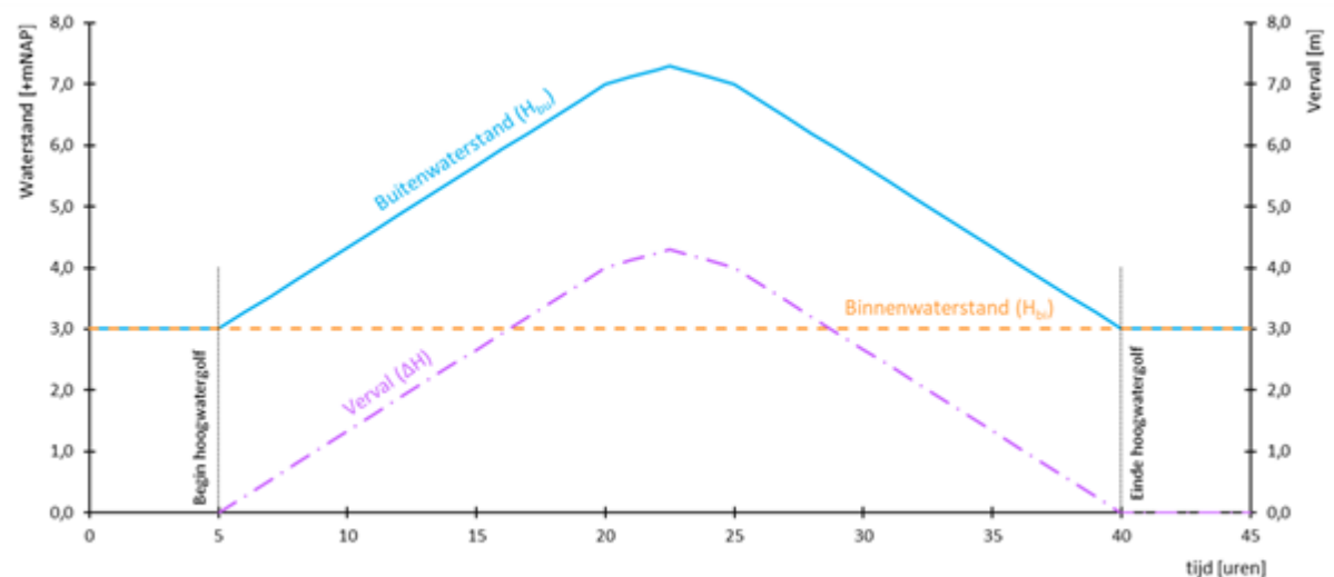
Figuur 3 Verval en binnenwaterstand bij hoogwater met constante buitenwaterstand en relatief grote komberging.
