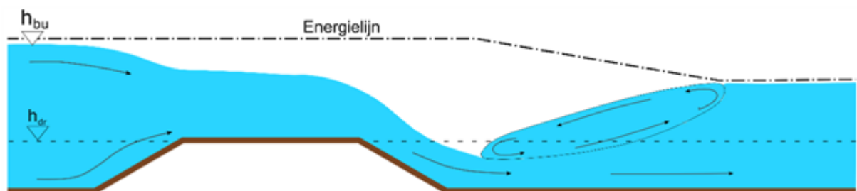
Figuur 1 Volkomen overlaat.
