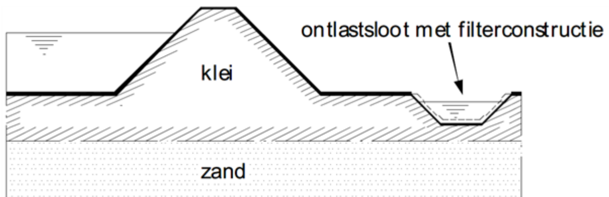
Figuur 1: Ontlastslot met filter.
