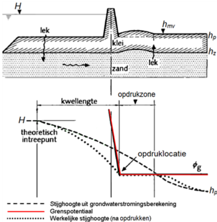
Figuur 1 Dijk met voorland en ondergrond. Stijghoogte in zandlaag, grenspotential en opdrukzone
