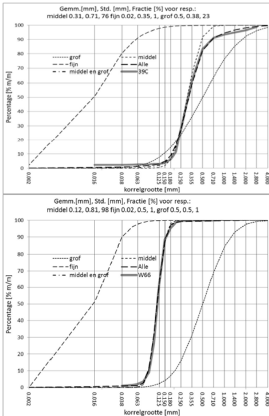
Figuur 4 Voorbeelden van korrelgrootteverdelingen van grondmonsters en van de daarin aanwezige fijne, middel en grove fracties. Het laatste monster betreft een getijdensandafzetting (B41-33, Waddenzeegebied).
