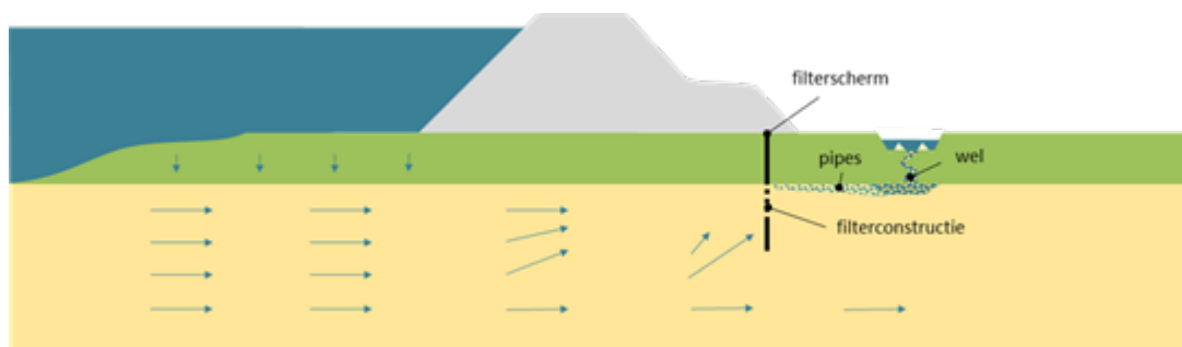
Figuur 4: Schematische weergave van de werking van een filterscherm.
