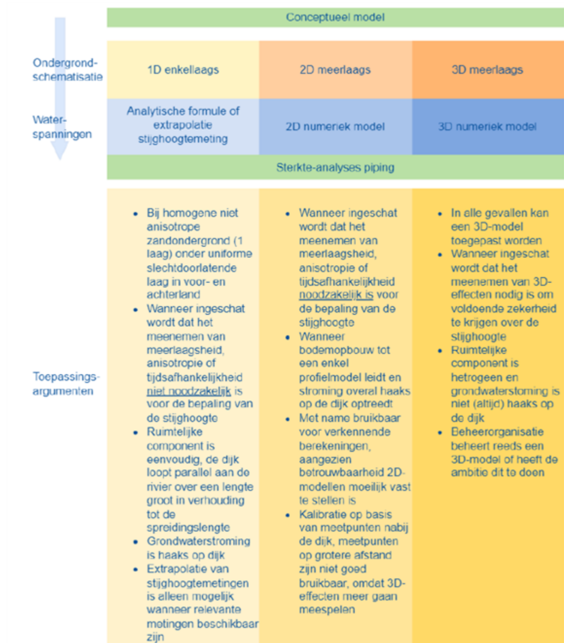
Figuur 1: Schema keuze methode vaststellen waterspanningen [Brinkhuis, et al., 2025]
