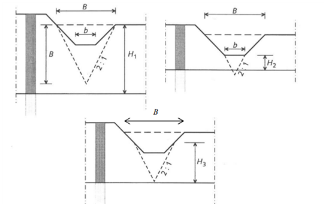
Figuur 1: Bepaling effectieve laagdikte voor opdrijven bij sloot
