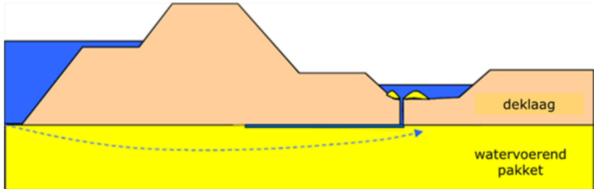
Figuur 1 Ontstaan van een terugschrijdend erosiekanaal
