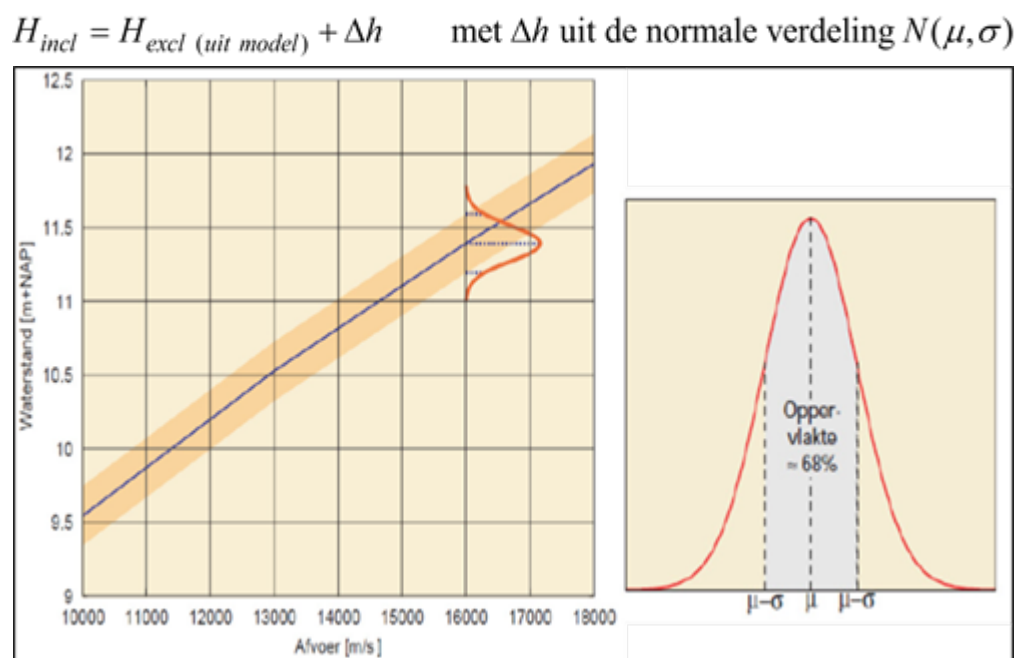
Figuur 1 Illustratie van onzekerheid in waterstand (als functie van stochast afvoer). In de linker figuur is een 95% betrouwbaarheidsband van 1 m aangehouden: 0,5 m hoger en 0,5 m lager voor het hele bereik.
