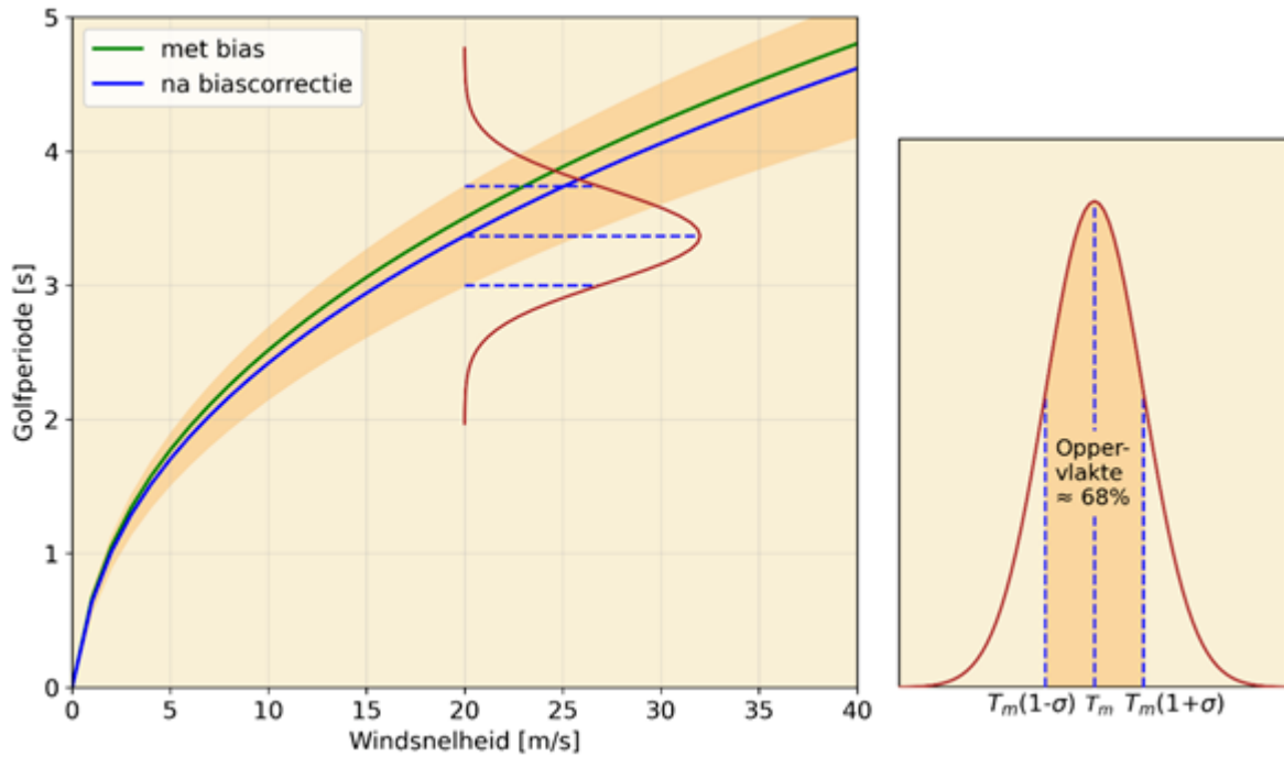
Figuur 2 Illustratie van de onzekerheid in de golferiode (als functie van de windsnelheid)
