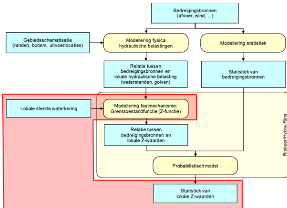
Figuur Stroomschema met positionering van de inzet van een speciale Z-functie ten behoeve van rekenwaarden voor de hydraulische belasting parameters.
