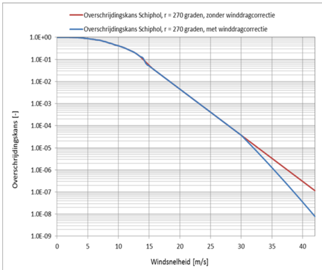
Figuur 1 Relatie windsnelheid en overschrijdingskans voor station Schiphol, 16 richtingssectoren, periode van 12 uur: met winddrag correctie (blauw) en zonder (rood).
