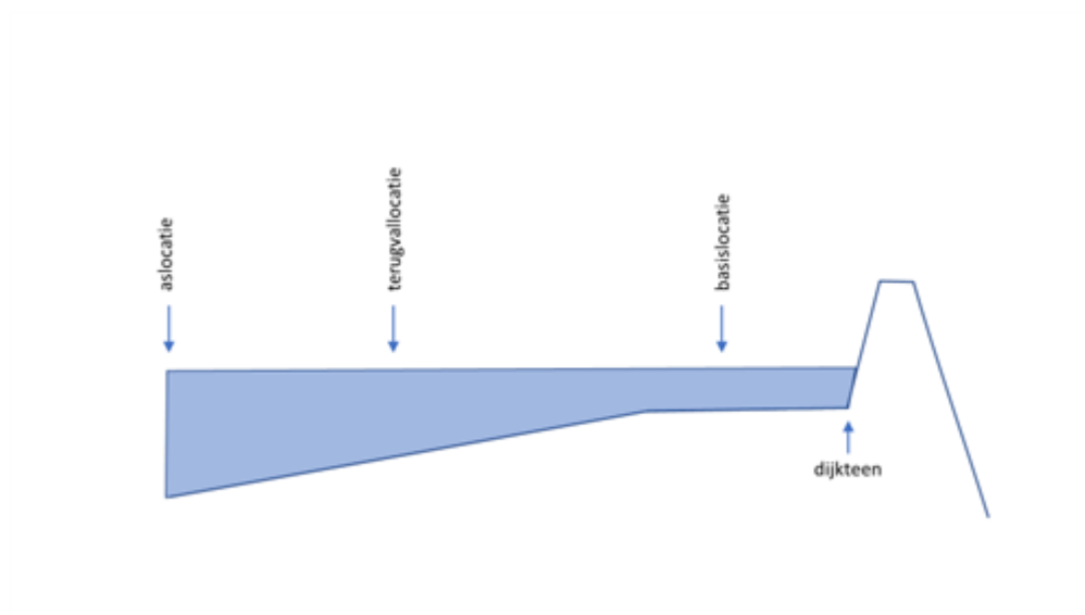
Figuur 2a Eerste voorbeeld positie van verschillende uitvoerlocaties ten opzichte van de dijkteen.
