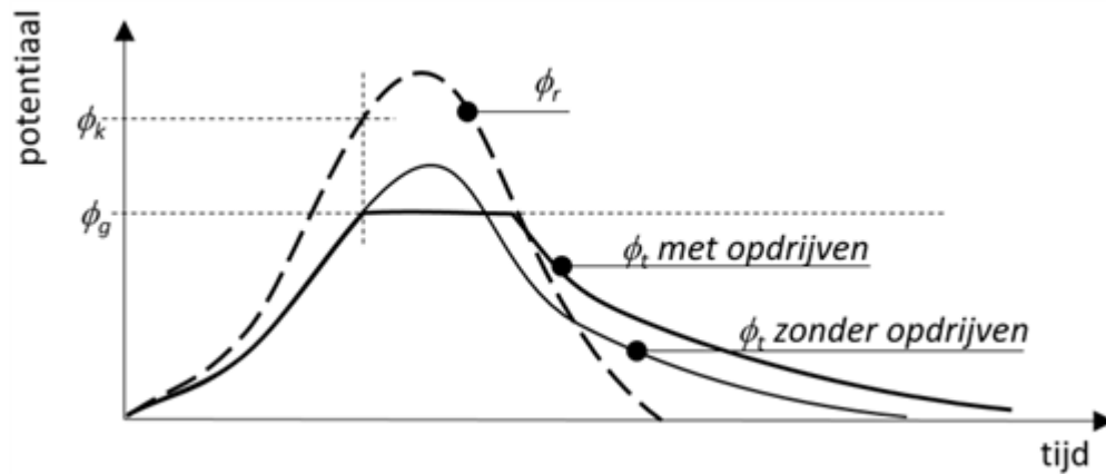
Figuur 1 Waterspanningsverloop in watervoerende laag bij opdrijven; \phi_r : stijghoogte peilbuis buitendijks (rivier), \phi_t : stijghoogte peilbuis binnendijks.
