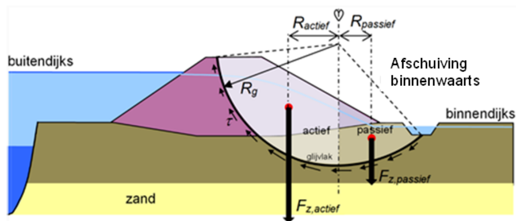
Figuur 1 Evenwichtsbeschouwing bij afschuiving binnenwaarts
