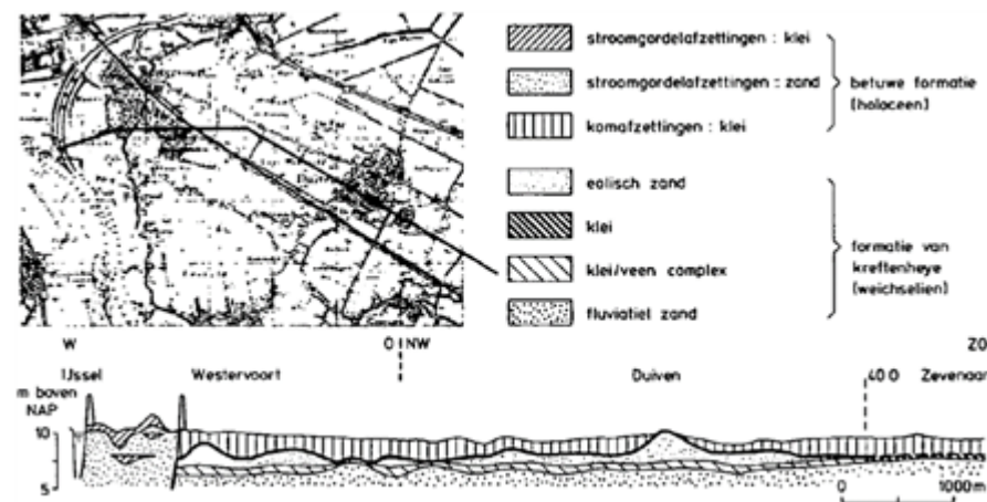
Figuur 2 Dwarsprofiel van het Komgebiet van de Westelijke Liemers (Ontleend aan de Geologische kaart van Nederland 1 :50.000, kaartblad Arnhem Oost (40 O) van de Rijks Geologische Dienst)
