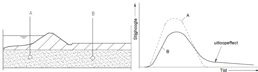
Figuur 1 Naijlen waterspanningen of uitloopeffect.
