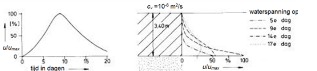
Figuur 2 Voorbeeld van aanpassing van de waterspanningen in een kleilaag (rechts), bij een gegeven drukgolf in de watervoerende zandlaag onder die kleilaag (links).
