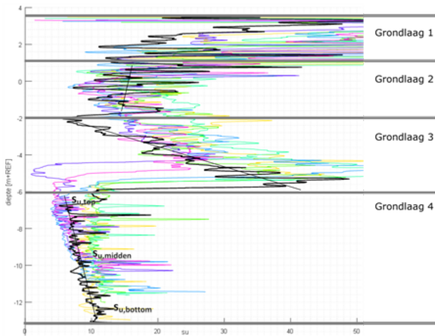
Figuur 1n de grondlagen 3 en 4 is een duidelijke trend over de diepte zichtbaar. De sterkte aan de bovenzijde van de lagen is beduidend lager dan aan de onderzijde en moet ook als zodanig gemodelleerd worden. Voor grondlaag 2 is het verschil tussen een lineair verloop of constante waarde niet significant.
