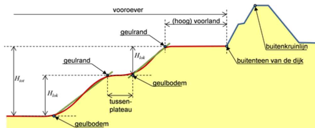
Figuur 1 Principeschets voorland met begrippen als de waterkering een dijk betreft.
