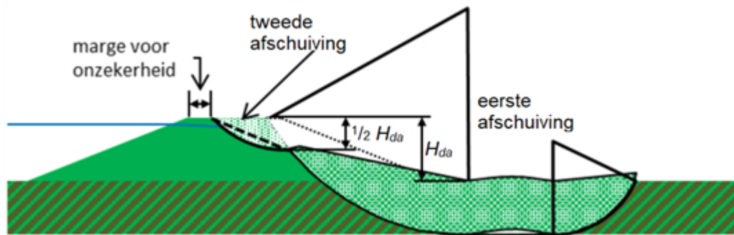
Figuur 1 Tweede afschuiving na eerste afschuiving.
