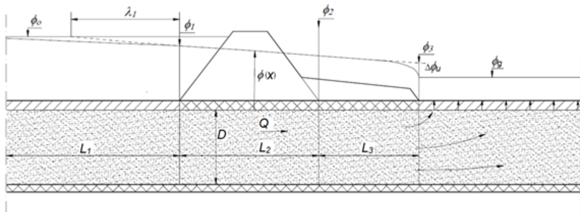
Figuur Optreden van de grenspotentiaal bij een situatie met een slecht doorlatende laag in het voorland
