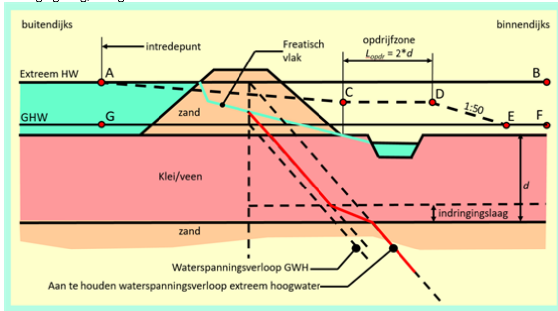
Figuur 2 Waterspanningen in wervoerend pakket voor geval 2A: zanddijk op ondoorlatende deklaag
