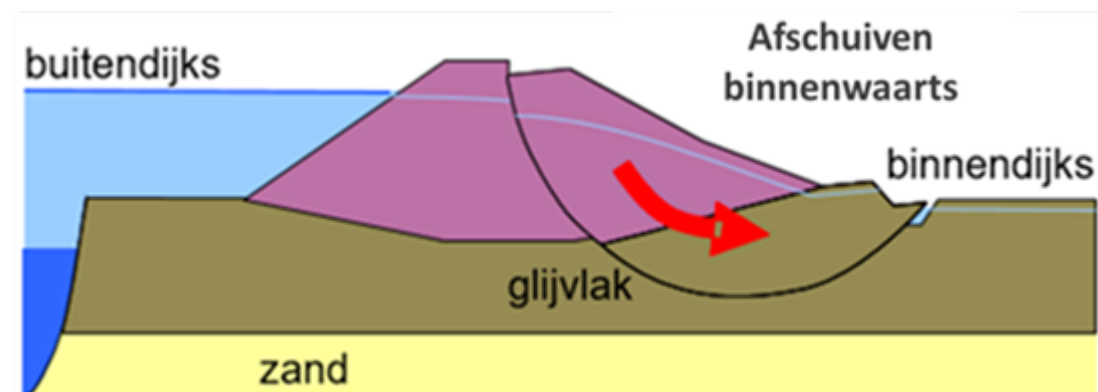
Figuur 1 Binnenwaartse afschuiving langs diep glijvlak.
