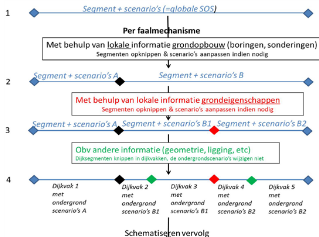
Figuur Processtappen vakindeling (generiek voor de mechanismen waarvoor de opbouw van de ondergrond relevant is). SOS-H is de SOS-Handleiding en de .
