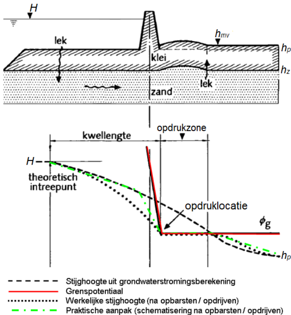
Figuur Dijk met voorland en ondergrond. Stijghoogte in zandlaag, grenspotential, opdrukzone en geschematiseerd waterspanningsverloop.
