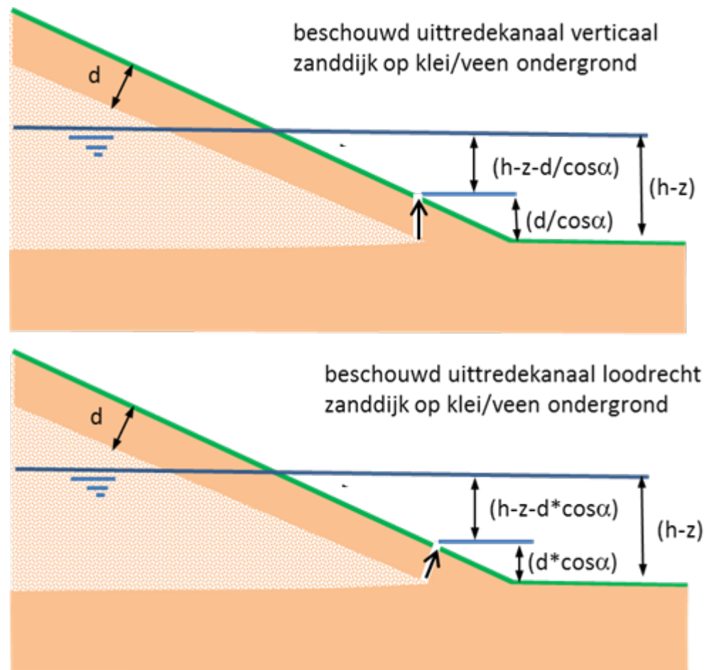
Figuur 1 Schematische weergave oriëntatie uittredekanaal met verval gegeven een grondwaterstand (h-z) in de zandkern, en de laagdikte van de kleilaag d .
