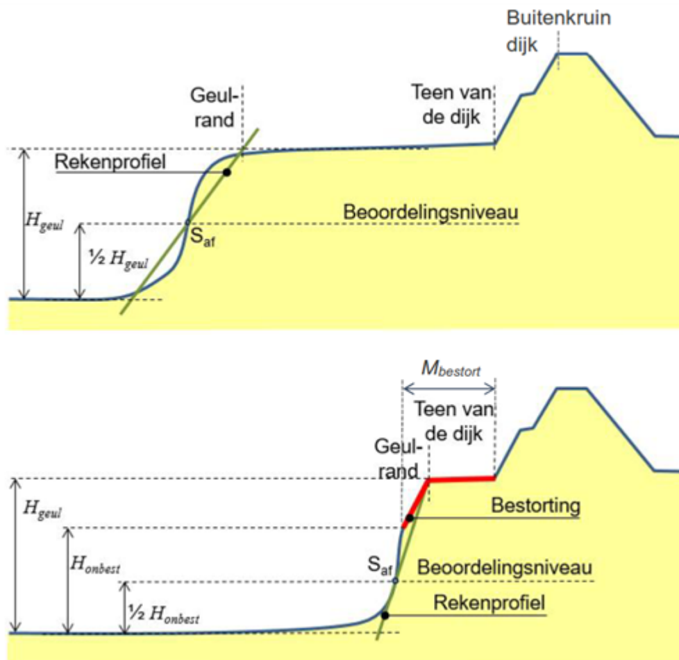
Figuur Definitie geschematiseerde geometrische parameters voor een situatie zonder bestorting (boven) en met bestorting (onder).
