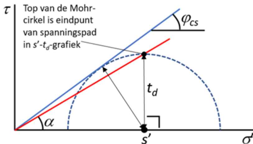
Figuur 2 Omrekening van de lijn door de toppunten van de Mohr-cirkel naar de lijn door de raakpunten van de Mohr-cirkels (de bezwijkomhullende)
