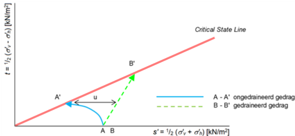
Figuur 1 Relatie tussen spanning s' en schuifsterkte t . De critical state line geeft de bezwijksterkte van de grond aan. De schuifsterkte bij punt B', uitgaande van gedraineerd grondgedrag, is duidelijk hoger dan de schuifsterkte bij punt A', uitgaande van ongedraineerd grondgedrag. De afstand u tussen de groene lijn en de blauwe lijn wordt veroorzaakt door de waterspanning.
