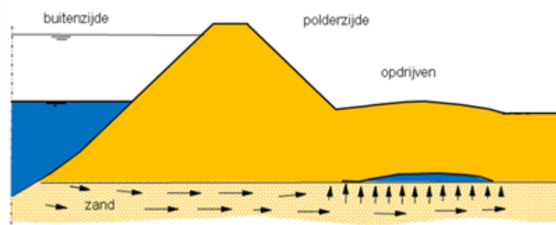
Figuur 2 Opdrijven.
