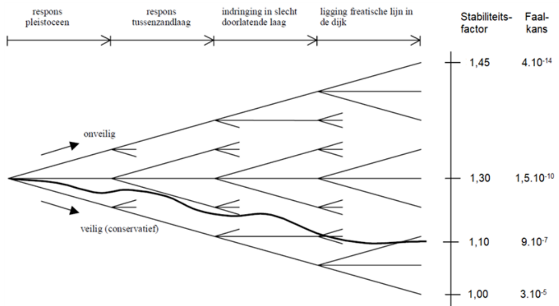
Figuur 2 (Fictieve) bandbreedte van de stabiliteitsfactor en bijbehorende faalkans als gevolg van door onzekerheden ingegeven keuzen bij de schematisering van waterspanningen
