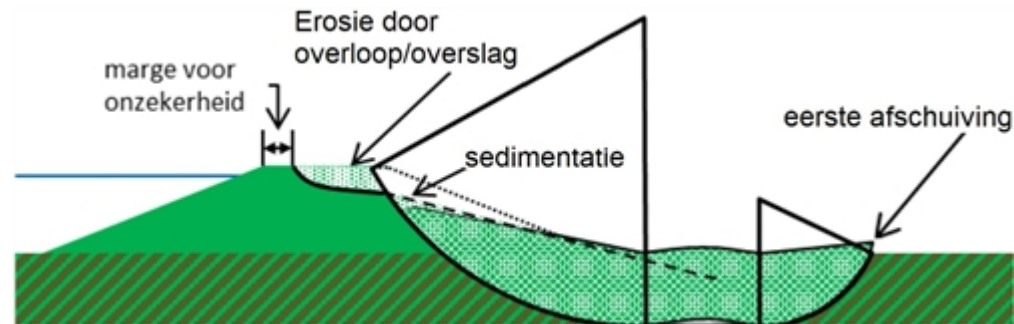
Figuur 1 Erosie door overloop/overslag na een binnenwaartse afschuiving.
