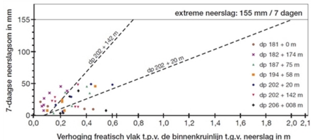
Figuur 1 Verband tussen gemeten freatische stijghoogtetoeenames (horizontaal) versus cumulatieve neerslag (verticaal) voor verschillende locaties langs een dijktraject aan de Lek in de buurt van Streefkerk [Swart, 1990]
