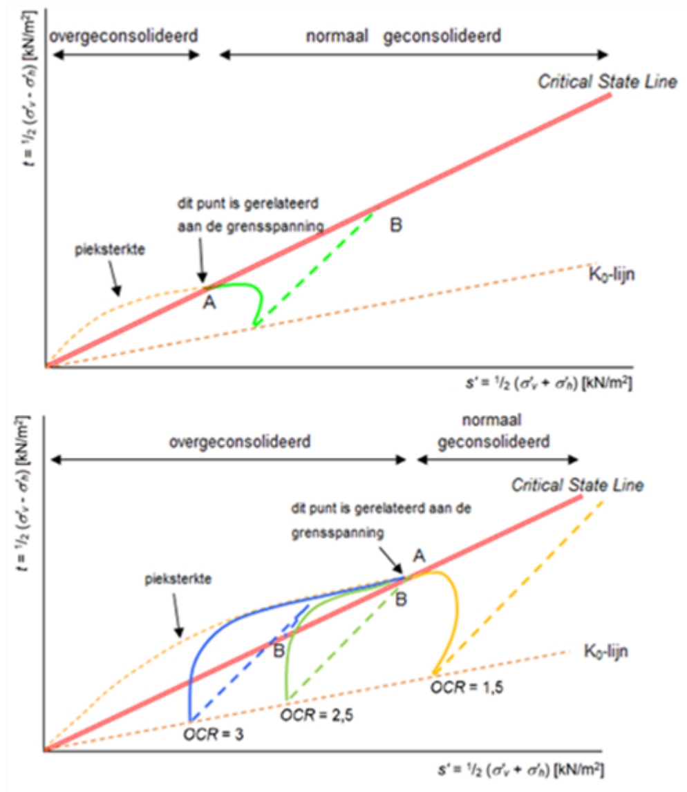
Figuur 2 Gedraineerd en ongedraineerd gedrag van grond weergegeven binnen het Critical State Soil Mechanics raamwerk. In de bovenste grafiek is de grond normaal geconsolideerd en vertoont de grond contractant gedrag ( OCR = 1 ) bij ongedraineerd afschuiven. In de onderste grafiek is de grond overgeconsolideerd en vertoont de grond contractant gedrag ( OCR < \approx 2,0 ) en dilatant gedrag ( OCR > \approx 2,0 ) bij ongedraineerd afschuiven
