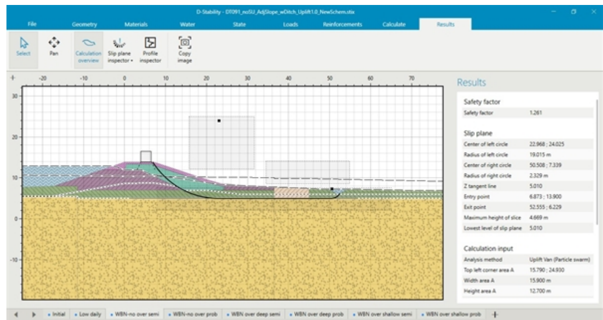
Figuur 2 Berekeningsresultaat van een berekening met het LiftVan-model met meerdere raaklijnen en met verwachtingswaarden en standaardafwijkingen van de ongedraineerde schuifsterkte op basis van de eindwaarde van triaxiaalproeven.
