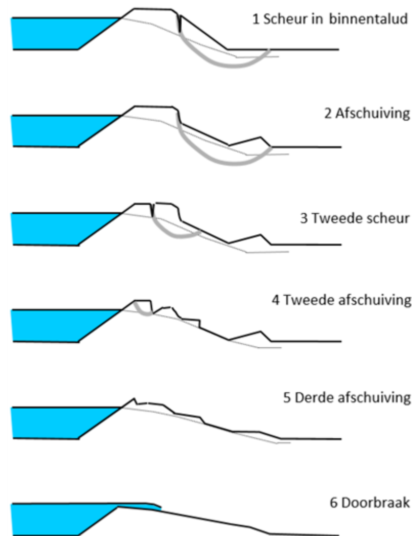
Figuur 3 Mogelijk faaltraject bij intredepunt schuifvlak in het binnentalud.
