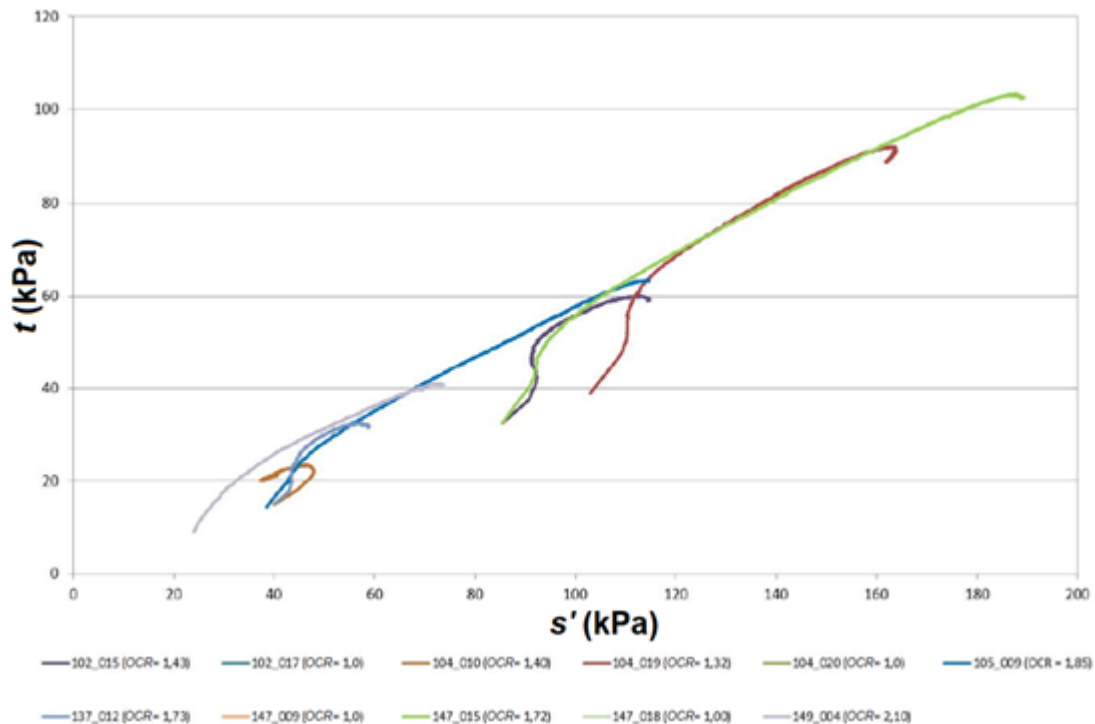
Figuur 1 Verloop van de schuifsterkte \tau_d als functie van de effectieve spanning s' voor een 11-tal zware zandige siltige kleimonsters uit het bovenrivierengebied. Voorbeeld van dilatant gedrag bij ongedraineerd afschuiven van siltige klei in het bovenrivierengebied.
