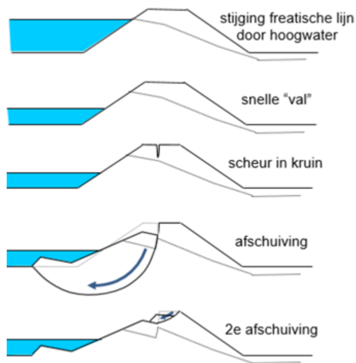
Figuur 3 Buitenwaartse afschuiving met intredepunt in de kruin.
