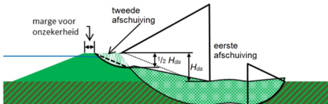
Figuur 1 Tweede afschuiving na eerste afschuiving.
