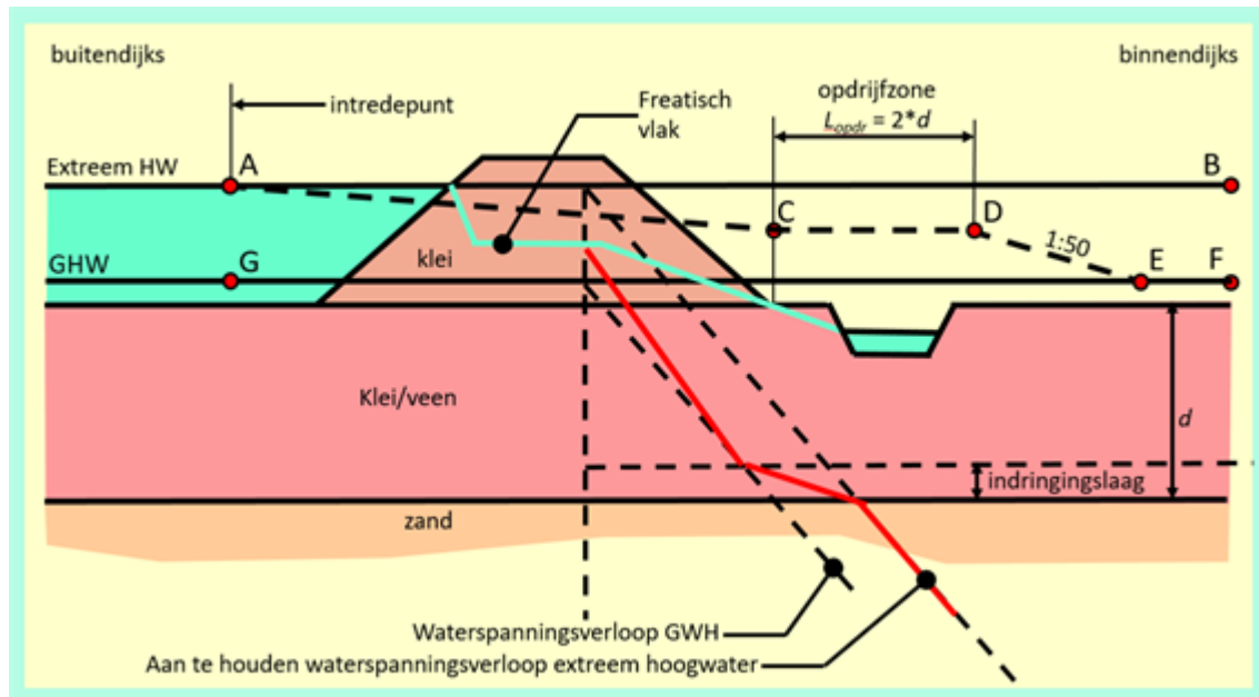
Figuur 1 Waterspanningen in watervoerend pakket voor geval 1A: kleidijk op ondoorlatende deklaag
