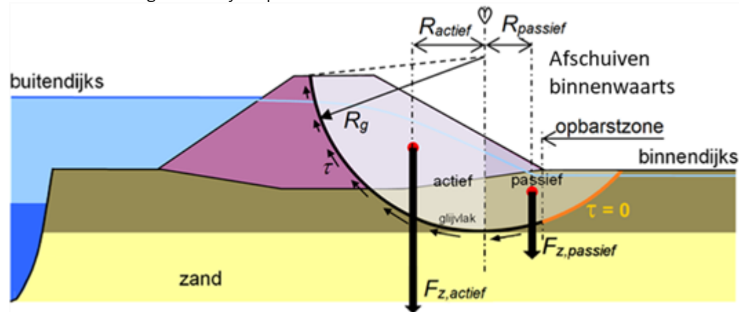
Figuur 1 Conservatieve schematisatie bij opbarsten: glijcirkel met schuifsterkte nul in de zone binnendijks van de teen.
