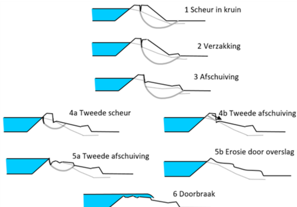
Figuur 2 Mogelijk faaltraject bij intredepunt schuifvlak in de kruin.
