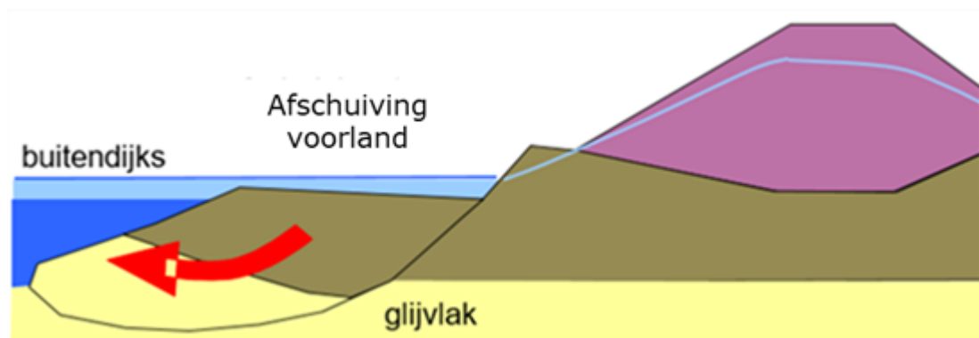
Figuur 1 Principeschets van het mechanisme afschuiven langs een glijvlak voorland.
