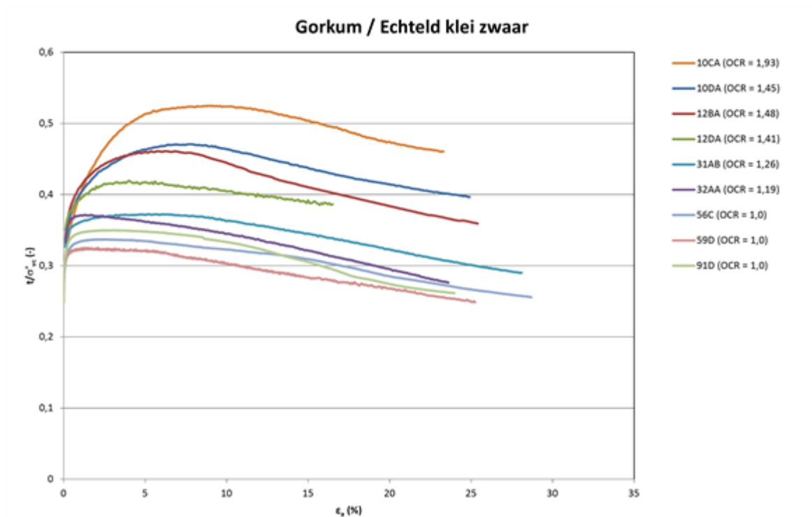
Figuur 1 Ratio t_d/\sigma'_{vc} of s_u/\sigma'_{vc} uitgezet tegen de axiale rek \epsilon_a
