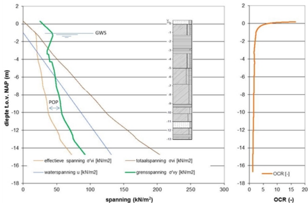
Figuur Totaalspanning \sigma'_{vi} , waterspanning u , effectieve verticale spanning \sigma'_{vi} en grensspanning \sigma'_{vy} (links) en de OCR (rechts) als functie van de diepte, in een grondprofiel.
