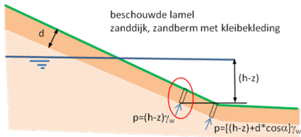
Figuur 2 Beschouwde lamel loodrecht evenwicht (afdrukken).
