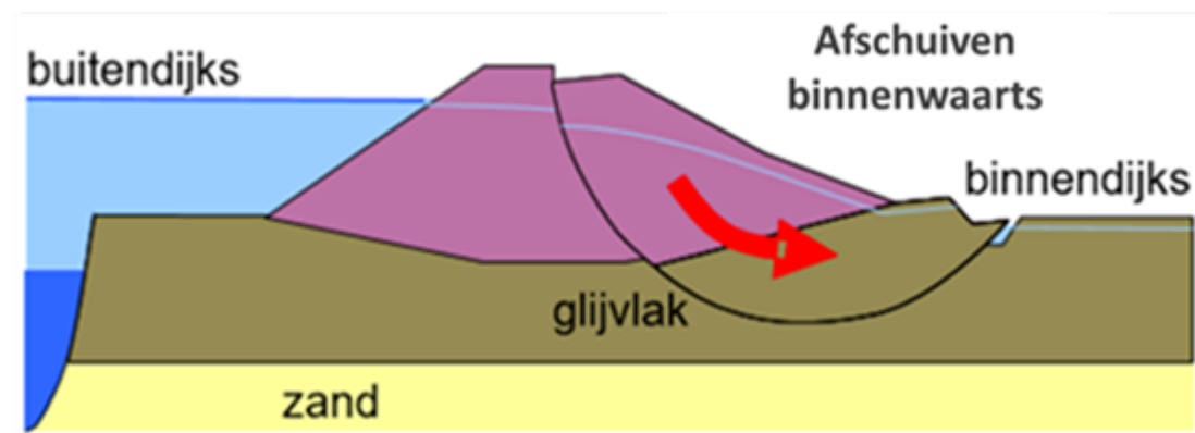
Figuur 1 Binnenwaartse afschuiving langs diep glijvlak.
