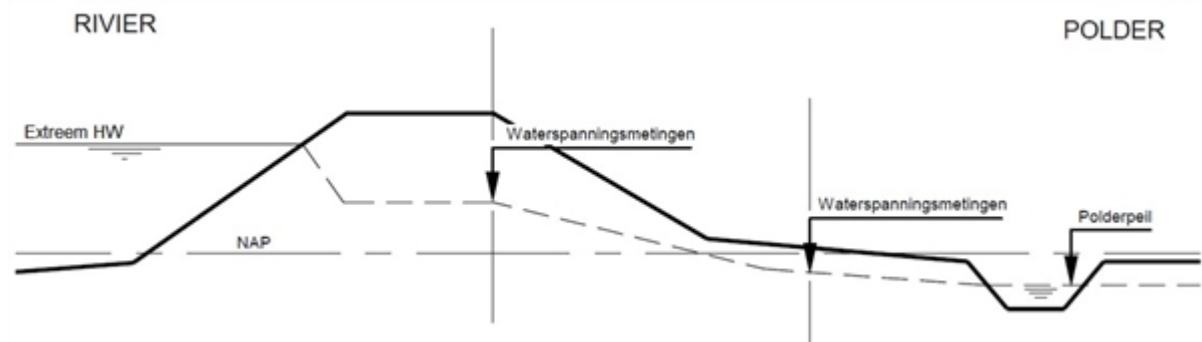
Figuur 2 Freatische lijn bij optreden extreem hoog water voor een rivierdijk met kleikern
