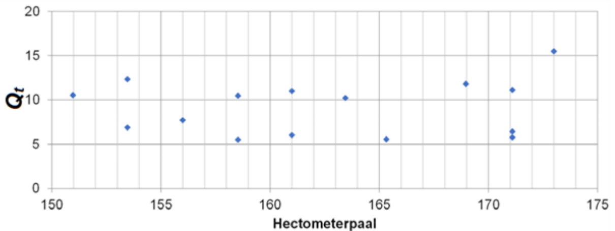
Figuur 5 Voorbeeld van het verloop van Q_t over een dijkvak, waarbij er geen trend is.
