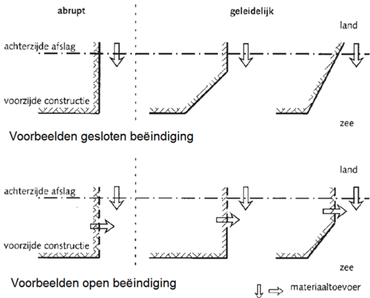
Figuur 1 Type beëindiging dijk in duin (boven: gesloten beëindiging, onder: open beëindiging).
