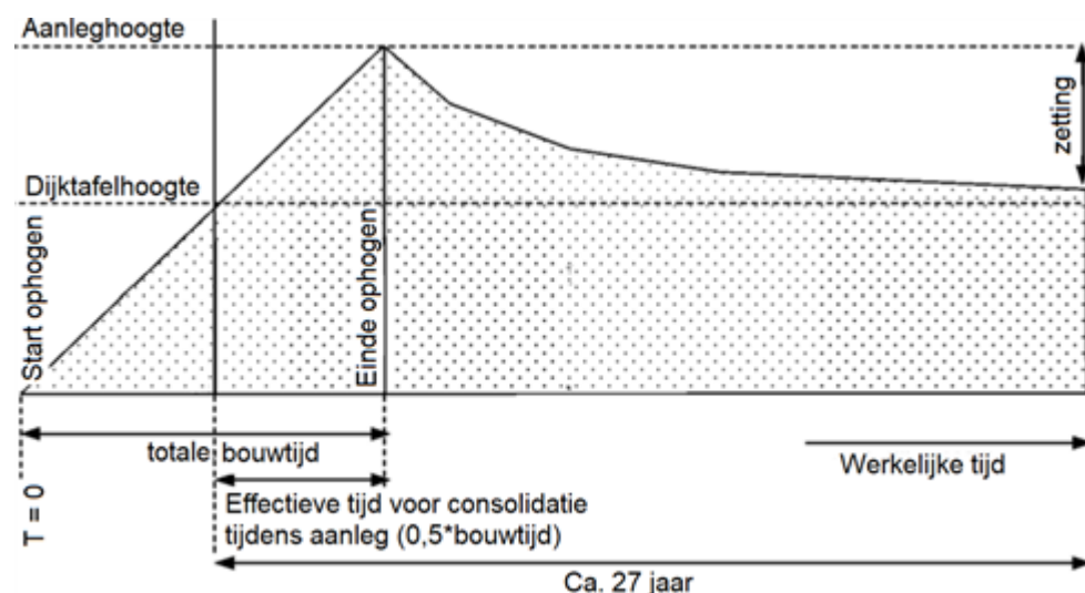
Figuur Dijkhoogte als functie van de tijd na de start van de uitvoering
