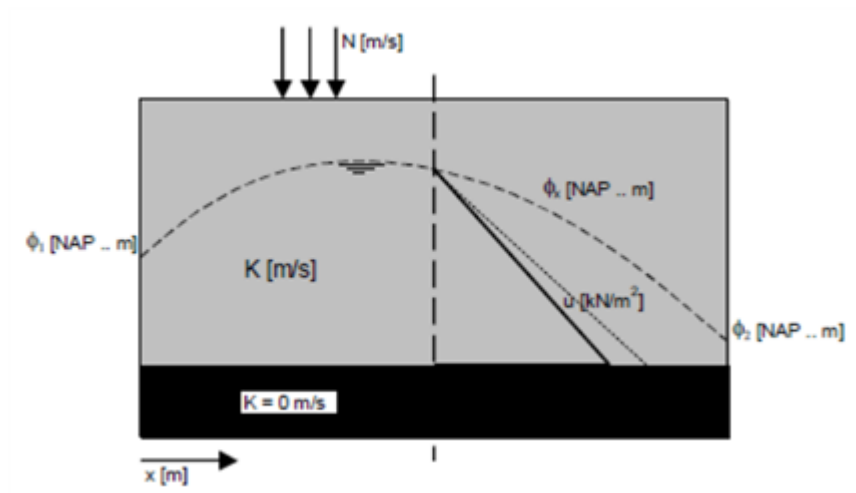
Figuur 1 Standaard-situatie waarvoor met de formule van Dupuit het niveau van het freatisch vlak is berekend. Het verloop van de waterspanning tegen de diepte is in een verticaal aangegeven.
