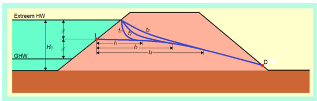
Figuur 2 Stijging van het freatisch vlak als gevolg een stijging van de buitenwaterstand en de daarbij behorende indringingslengte. NB, de in deze figuur weergegeven verlopen van de freatische lijn zijn realistischer dan het meer geschematiseerde verloop in figuur 1.
