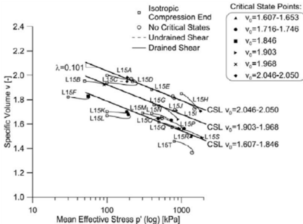
Figuur 4 Voorbeeld van de ligging van de critical state line afhankelijk van het specifiek volume v van het materiaal. Siltige klei met 10 a 20% lutum van de lagunes bij Venetië [Ponzone, 2014]
