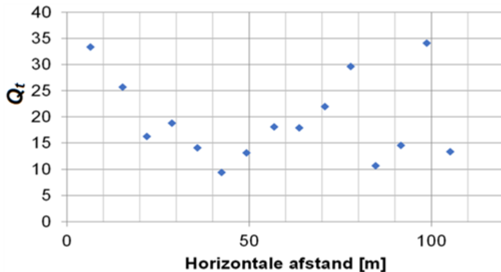
Figuur 6 Voorbeeld sondeerafstand 10 meter. Reken met een set aan sonderingen. Reken met het gemiddelde over het schuifvlak, breng uitmiddeling over de breedte in rekening. ( \gamma=0,0 \text{ á } 0,25 ).
