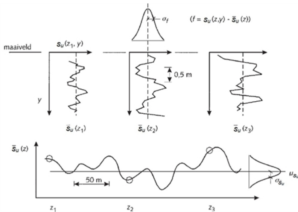
Figuur 1 Mogelijk variatiepatroon van ongedraineerde schuifsterkte in een slappe kleilaag
