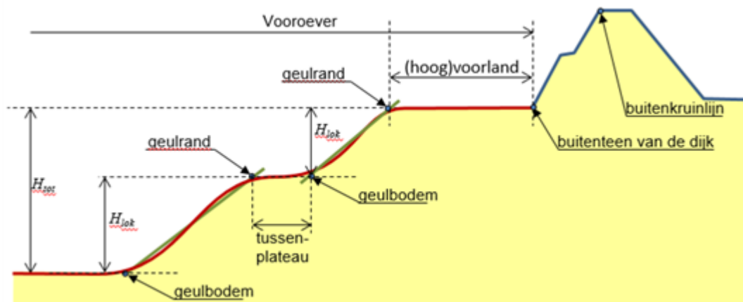
Figuur 2 Principeschets voorland met een tussenplateau.
