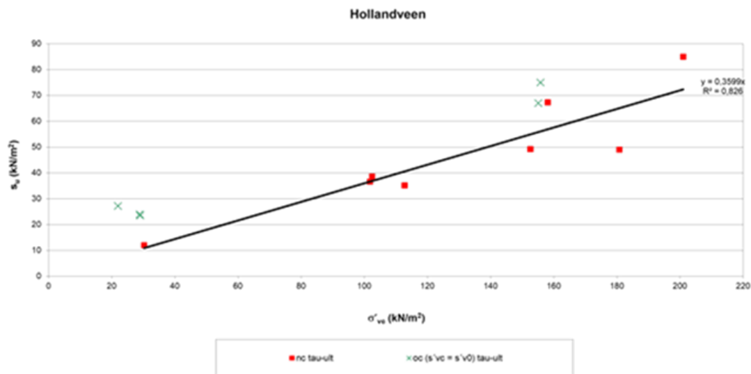
Figuur 4 Schuifsterkte s_u uit de direct simple shear proeven op Hollandveen uitgezet tegen de consolidatiespanning \sigma'_{vc} van de DSS proeven; waarden bij 40% schuifrek.
