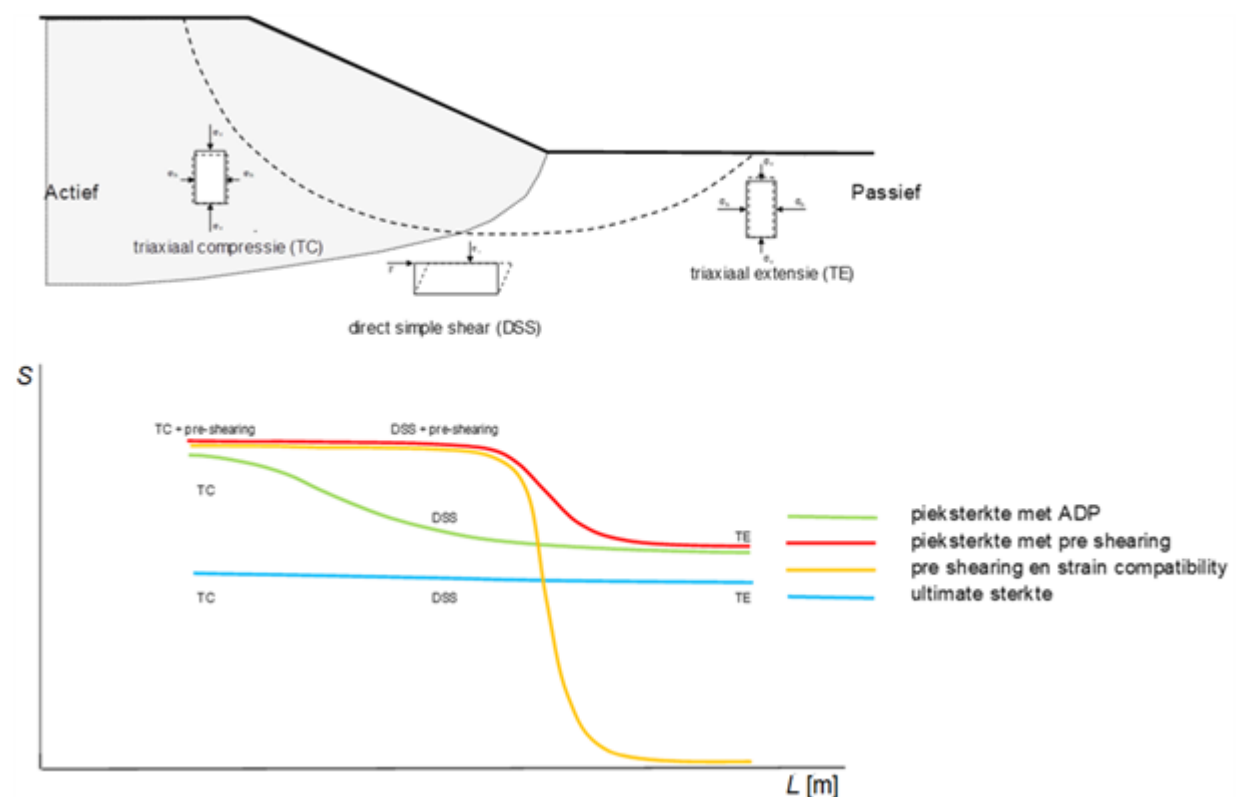
Figuur 2 Schematische weergave van de ongedraineerde schuifsterkte ratio S langs het schuifvlak met effecten van anisotropie, pre shearing, softening en strain compatibility
