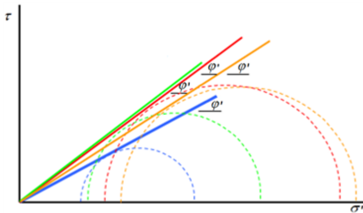
Figuur 3 De hoeken van inwendige wrijving \varphi'_{cs} van meerdere triaxiaalproeven worden bij elkaar genomen om een verwachtingswaarde en standaardafwijking van de hoek van inwendige wrijving te bepalen
