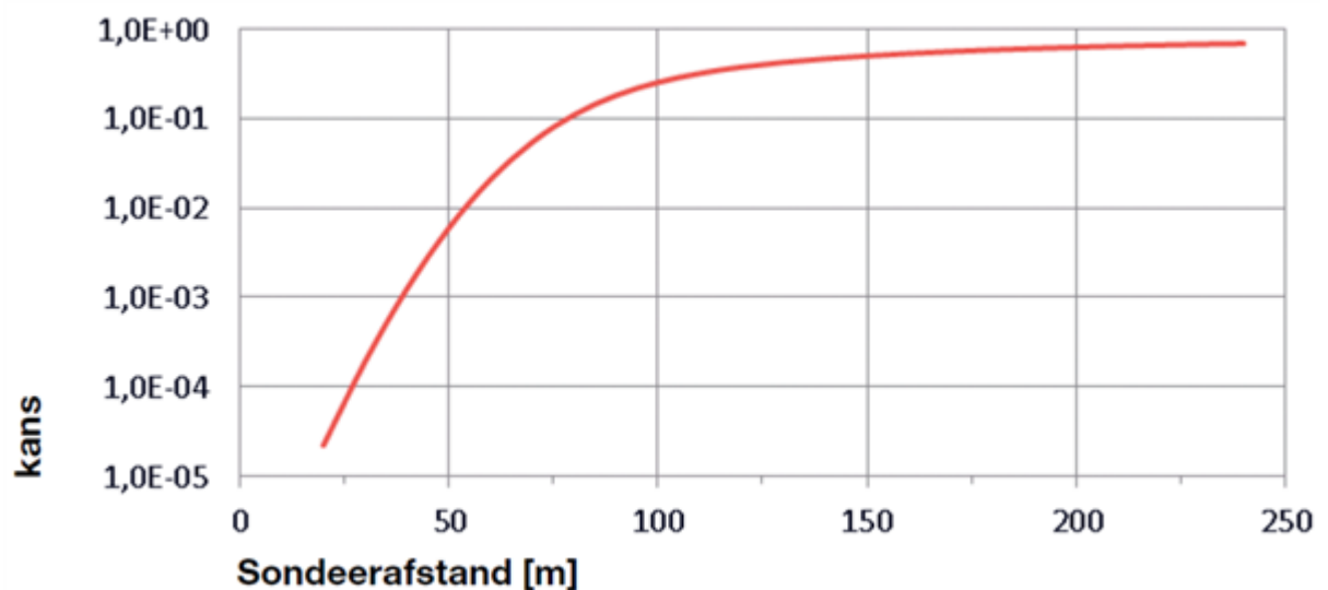
Figuur 1 Kans op 'missen' van een lens met slap bodemmateriaal als functie van de sondeerafstand bij equidistante sonderingen. Ontleend aan [Calle, 2002]
