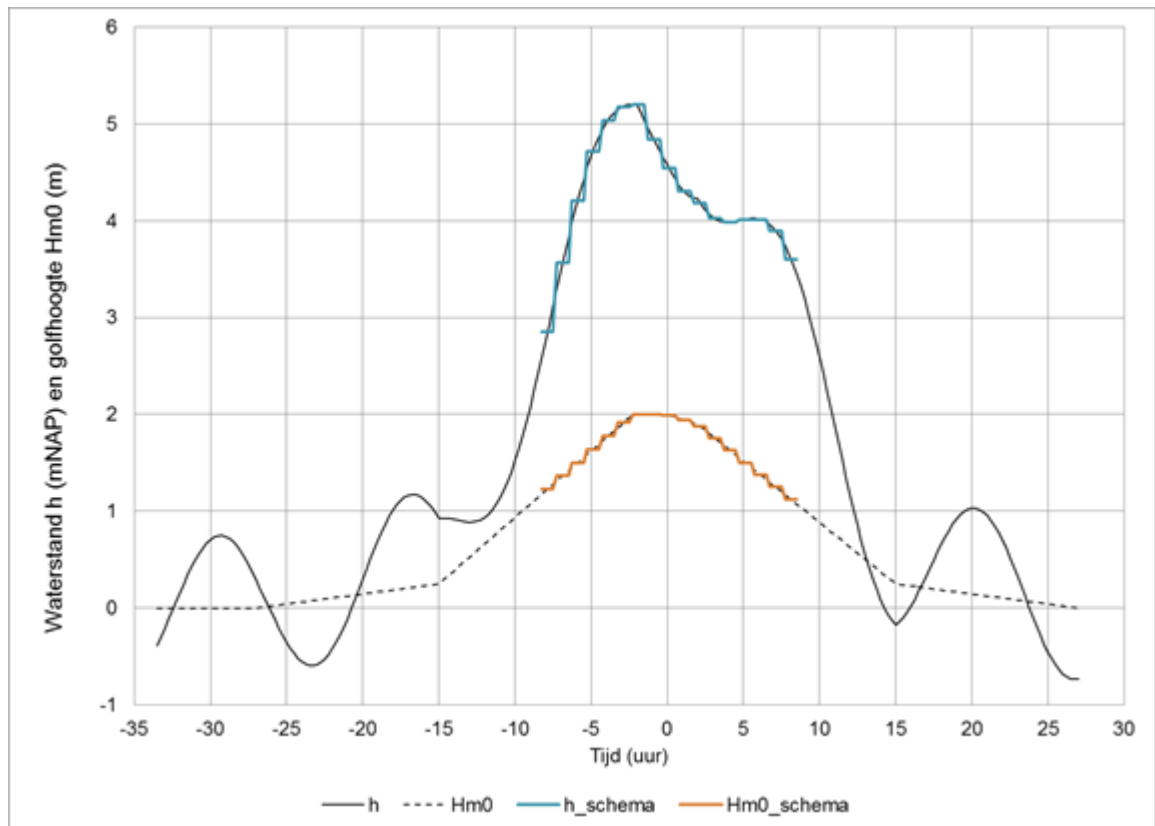
Figuur 2 Verloop in tijd van de significante golfhoogte H_{m0} [m] en de buitenwaterstand h [m] en de schematisering hiervan in discrete stukjes van 1 uur [RWS 2016a]
