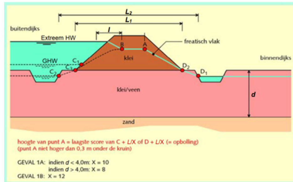
Figuur 1 Freatisch vlak voor de gevallen 1A en 1B
