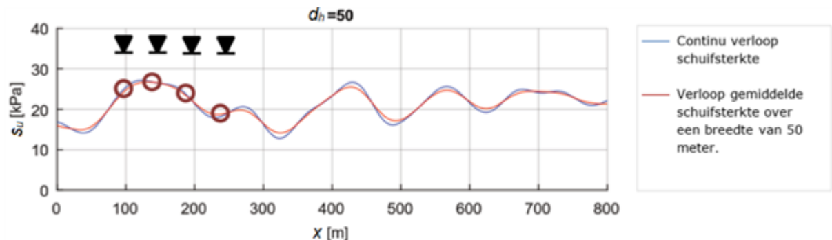
Figuur 1 Bij correlatielengtes in de orde van 50-150 meter geven afzonderlijke sonderingen met een tussenafstand van 50 meter (rode cirkels) een goed beeld van de sterkte die over de breedte van een potentieel afschuifvlak in de ondergrond aanwezig is (rode lijn).
