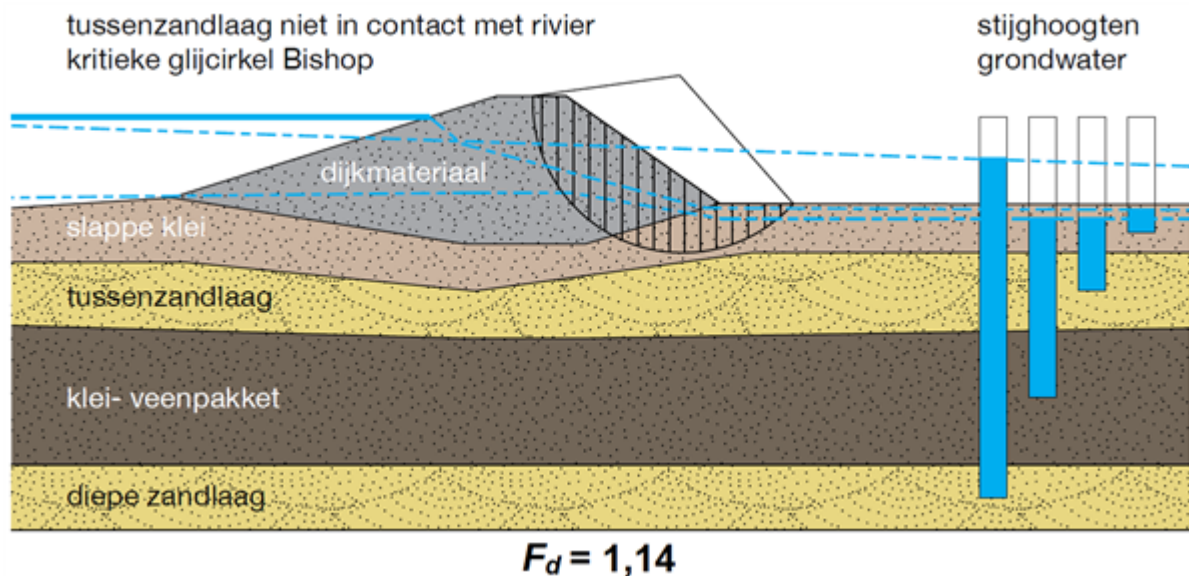
Figuur 1 Schematisering van de opbouw van een dijk en de ondergrond voor de controle op het mechanisme afschuiven
