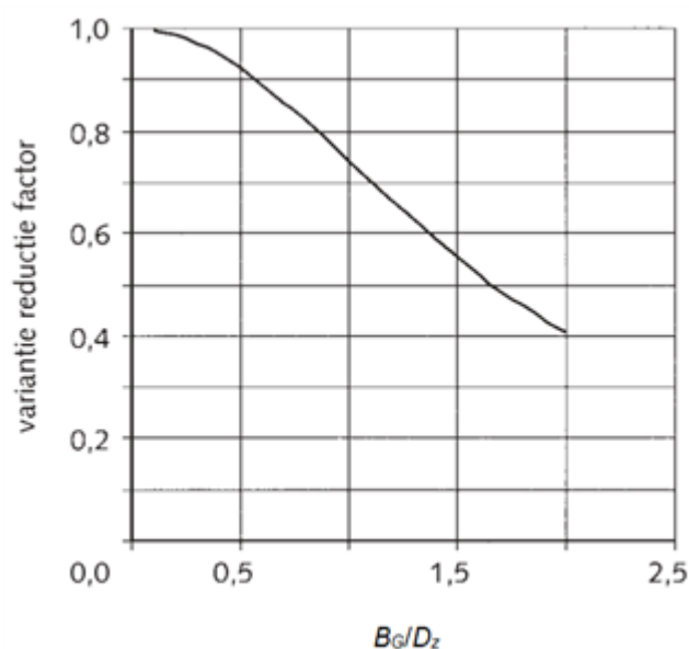
Figuur 2 Variantiereductiefactor voor uitmiddeling in horizontale richting
