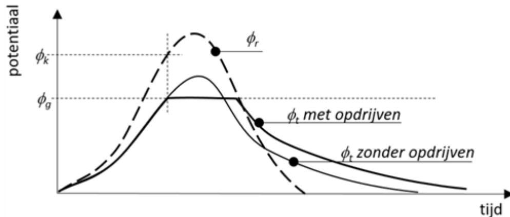
Figuur 1 Waterspanningsverloop in watervoerende laag bij opdrijven; \phi_r : stijghoogte peilbuis buitendijks (rivier), \phi_r : stijghoogte peilbuis binnendijks.
