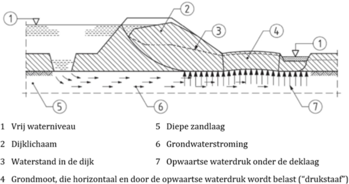
Figuur 4 Schuifvlak bij opdrijven van het achterland met glijvlak naar het maaiveld (= slootbodembodem).
