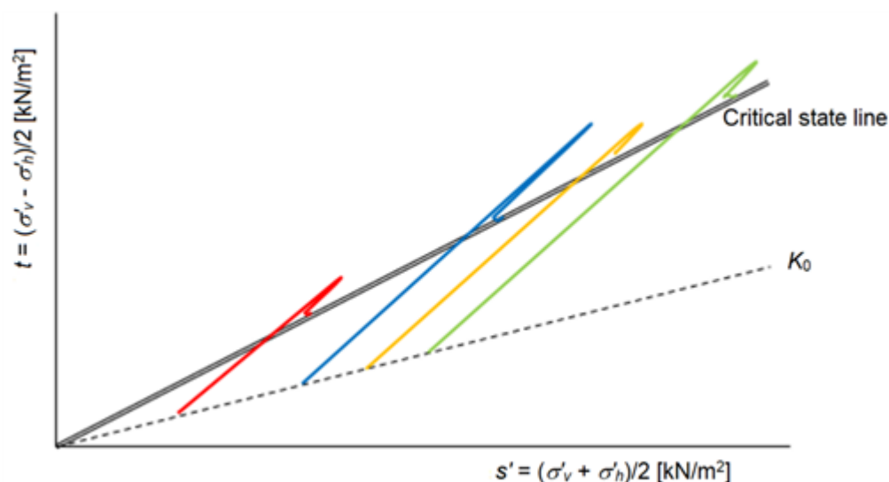
Figuur 1 Grafiek waarin de halve deviatorspanning t tegen het gemiddelde van de hoofdspinningen s' is uitgezet. Hierin staan spanningspaden uit gedraineerde triaxiaalproeven. De Critical State Line gaat door de s' - en t -waarden bij het einde van de proeven en door de oorsprong van de grafiek
