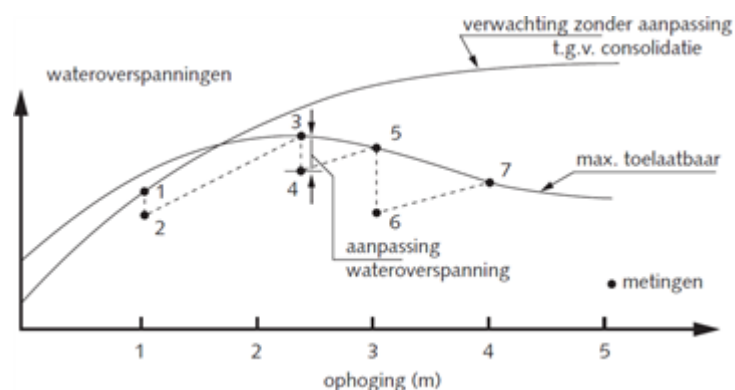
Figuur Verwachte wateroverspanning als functie van de ophoging
