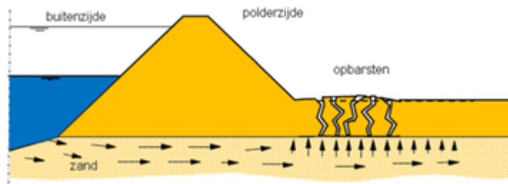
Figuur 3 Opbarsten.
