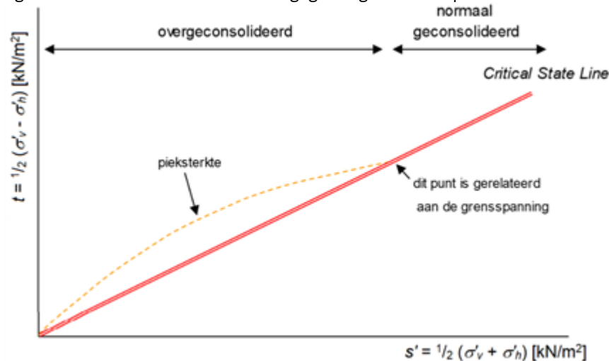
Figuur Karakterisering van de schuifsterkte volgens het Critical State Soil Mechanics raamwerk (CSSM)
