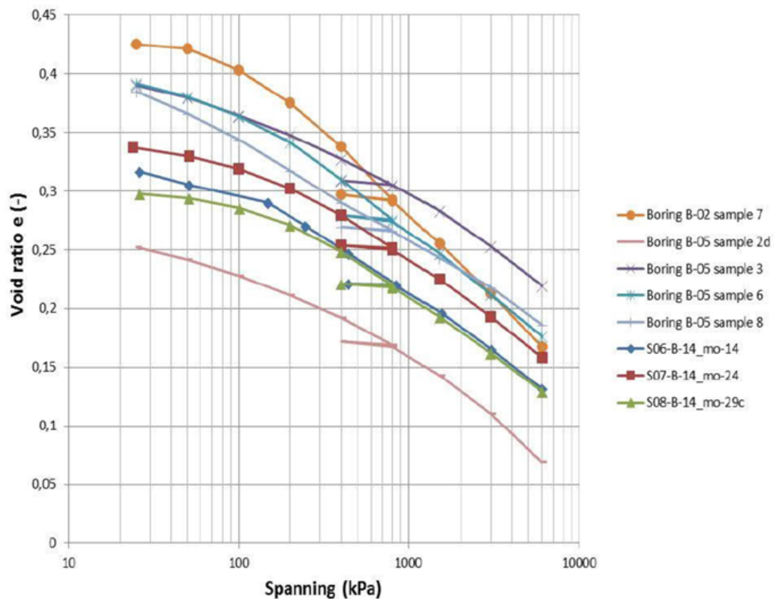
Figuur 2 Voorbeelden van samendrukkingscurves van Keileem
