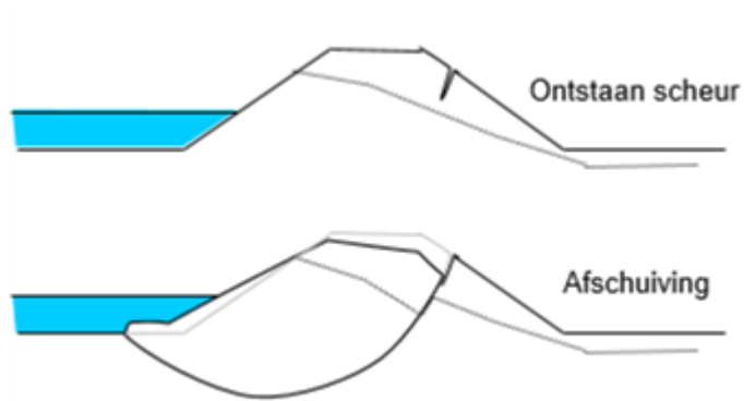
Figuur 4 Buitenwaartse afschuiving met intredepunt in het binnentalud.
