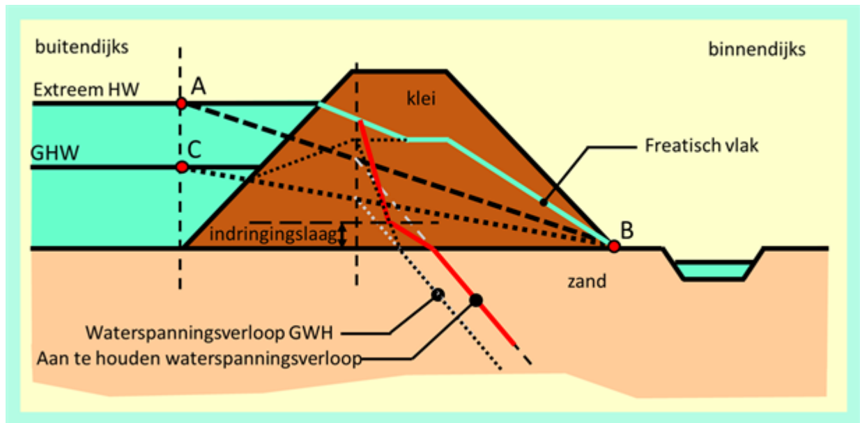
Figuur 3 Waterspanningen in het eerste watervoerend pakket voor geval 1B: kleidijk op zand, NB voor de ligging van de freatische lijn in de dijk, zie Eerste schatting van het freatisch vlak
