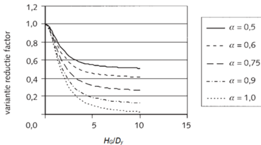
Figuur 3 Variantiereductiefactor voor uitmiddeling in verticale richting
