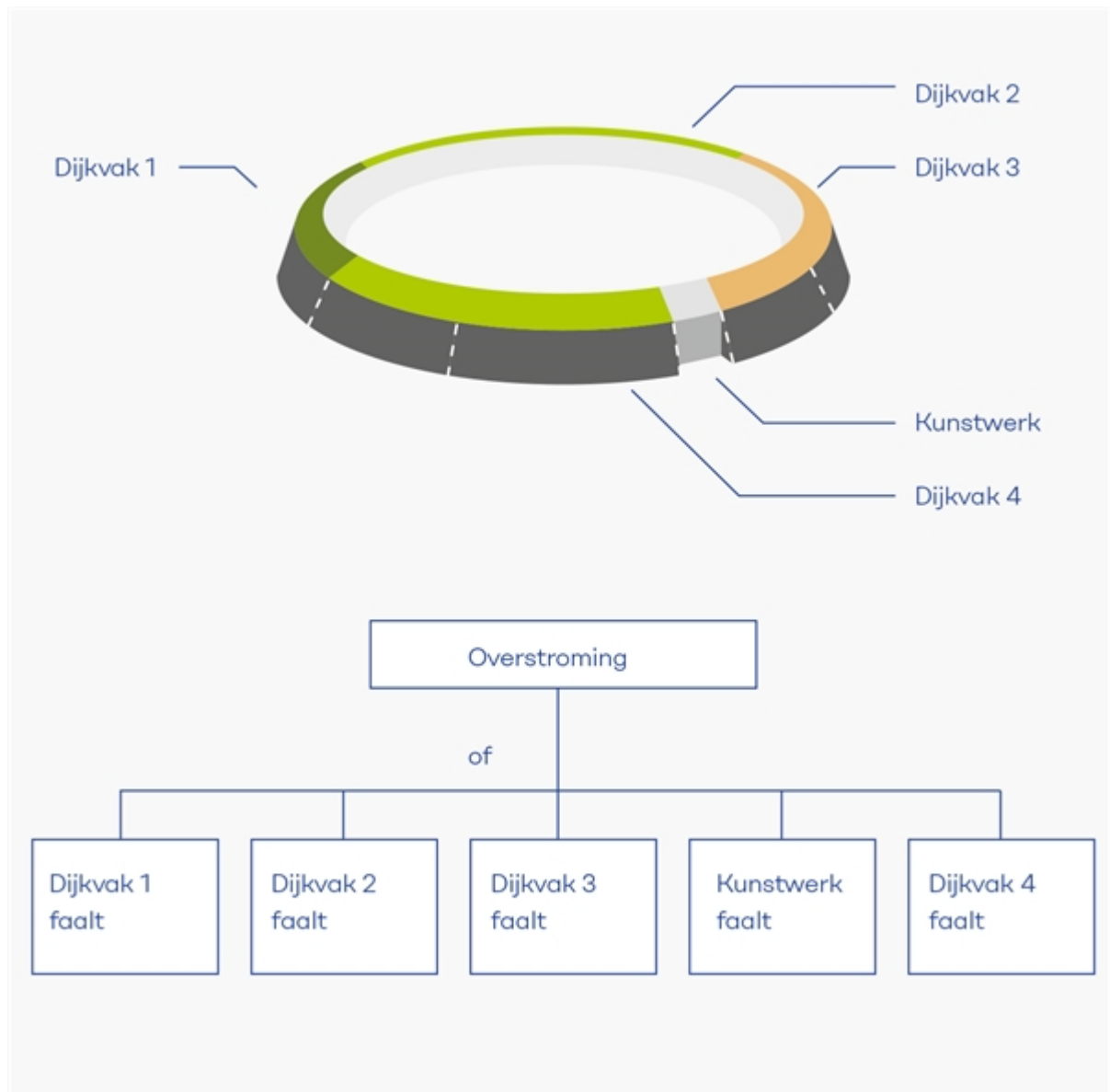
Figuur 1 Foutenboom.
