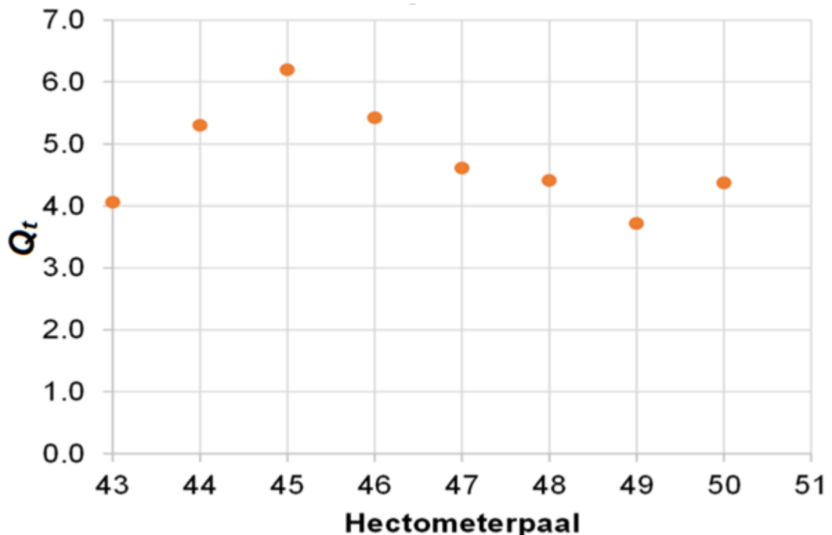
Figuur 4 Voorbeeld van het verloop van Q_t over een dijkvak. In dit geval moet de lokale sondering bij 43 of 49 gebruikt worden, omdat verondersteld wordt dat deze (minimale) sterkte over de breedte van een afschuifvlak aanwezig is.
