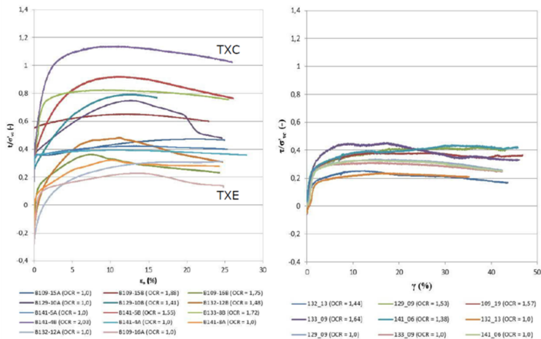
Figuur 5 Ongedraineerde schuifsterkte anisotropie bij siltige klei met triaxiaal compressie proeven (TXC) en triaxiaal extensie proeven (TXE) (links) en direct simple shear proeven (rechts)
