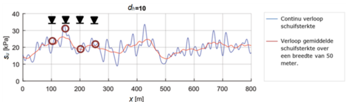
Figuur 2 Bij correlatielengtes die een orde kleiner zijn dan de breedte van een potentieel afschuifvlak, geven afzonderlijke sonderingen (rode cirkels) met een tussenafstand van 50 meter geen goed beeld van de gemiddelde sterkte die over de breedte van een potentieel afschuifvlak in de ondergrond aanwezig is (rode lijn).
