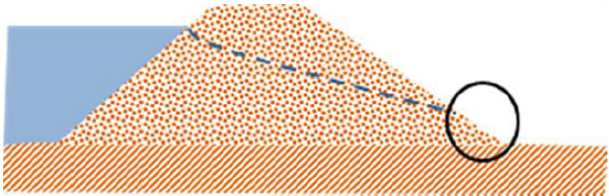
Figuur 3 Uitspoelen.
