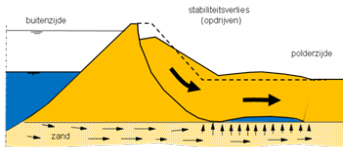
Figuur 5 Afschuiven binnentalud met opdrijven en vervorming achterland.
