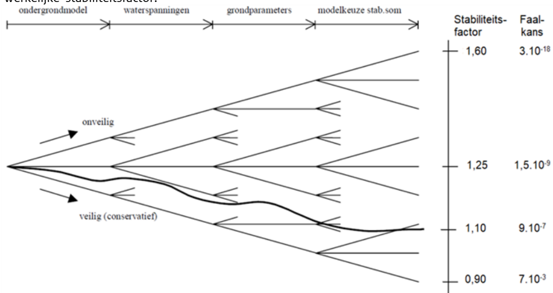
Figuur 1 Bandbreedte van berekende stabiliteitsfactor (mechanisme afschuiven langs een glijvlak binnenwaarts) en daarbij behorende faalkans als gevolg van door onzekerheden ingegeven mogelijke keuzen bij de schematisering (de getallenrange is fictief). De dikke lijn representeert een betrekkelijk veilige wijze van schematiseren volgens de inmiddels achterhaalde overbelastingsbenadering.
