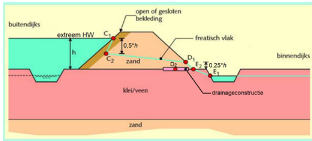
Figuur 3 Freatisch vlak voor geval 2A
