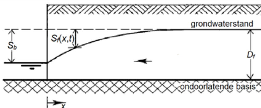
Figuur Tijdsafhankelijke, een-dimensionale grondwaterstroming in een semi-oneindig onbegrensde aquifer
