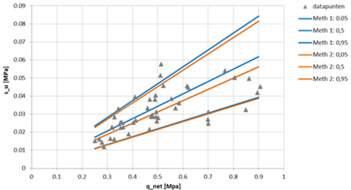
Figuur Voorbeeld: 90 % betrouwbaarheidsinterval voor s_u = q_{net}/N_{kt} weergegeven door de lijn voor de verwachtingswaarde en de lijnen voor de 5% over- en onderschrijdingswaarden van de N_{kt} . Getoond worden de resultaten volgens methode 1 ( N_{kt}=14,6 en VC(gem(q_{net}/N_{kt}))=0,22 ) en volgens methode 2 ( N_{kt}(p=0,05)=11,0 ; N_{kt}(p=0,5)=16,0 ; N_{kt}(p=0,95)=23,2 ).
