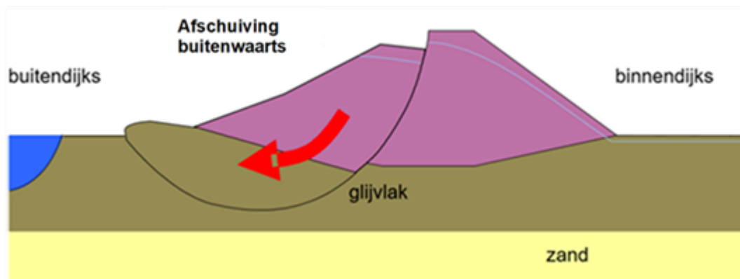
Figuur 1 Buitenwaarts afschuiven van het buitentalud
