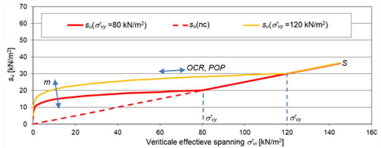
Figuur Relatie tussen ongedraineerde schuifsterkte en effectieve spanning volgens het SHANSEP-model, met de rol van de parameters S , m , OCR en POP
