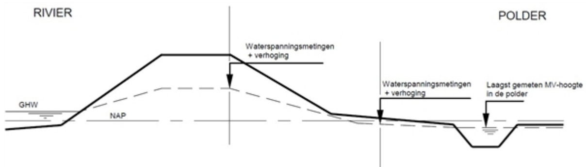
Figuur 3 Freatische lijn bij extreme neerslag
