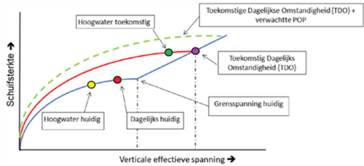
Figuur Overzicht ontwikkeling schuifsterkte onder dagelijkse en toekomstige omstandigheden
