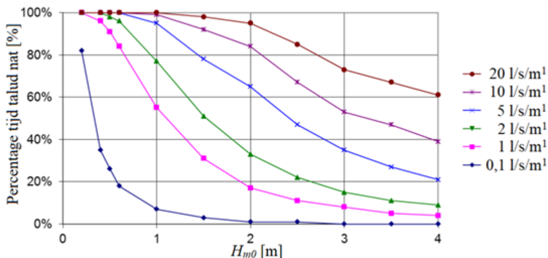
Figuur 1 Infiltratietijd als percentage van de beschouwde periode gegeven de significante golfhoogte H_{m0} [m] en het gemiddelde overslagdebiet q_g [l/s/m] [RWS 2016b]
