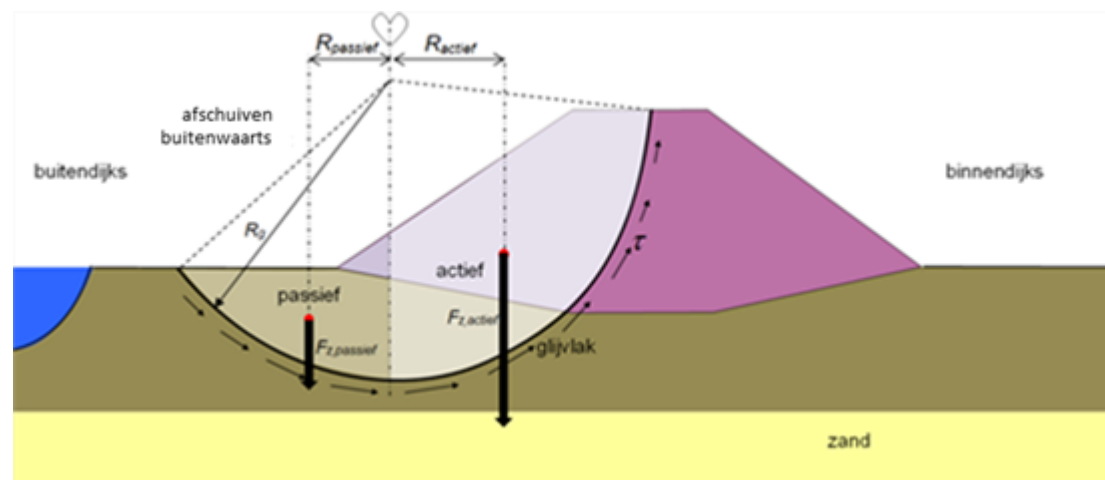
Figuur 2 Evenwichtsbeschouwing bij afschuiven buitentalud.
