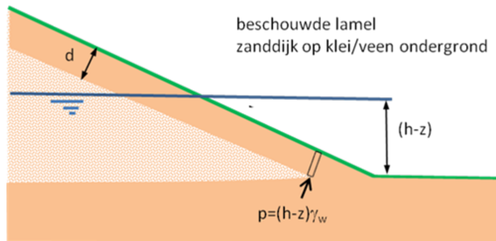
Figuur 1 Beschouwde lamel loodrecht evenwicht (afdrukken).
