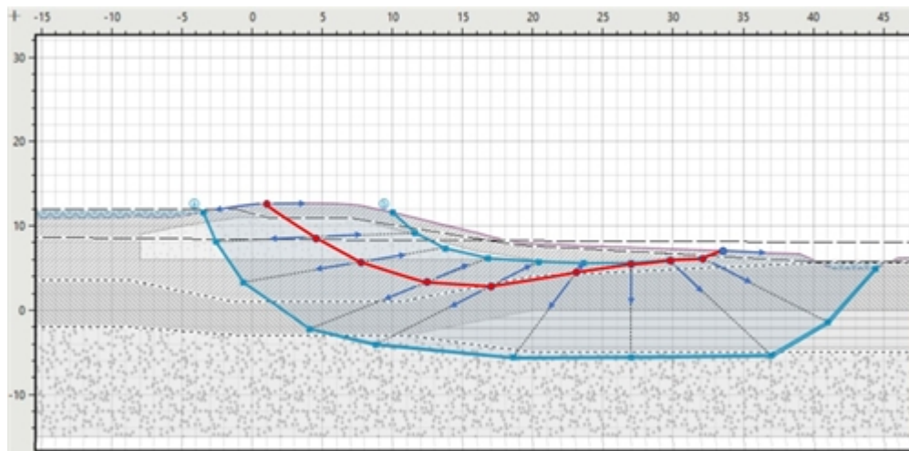
Figuur 2 De rode punten die het glijvlak beschrijven kunnen vrij bewegen langs de verbindinglijnen tussen de onder- en bovengrens, op zoek naar het meest kritische glijvlak.
