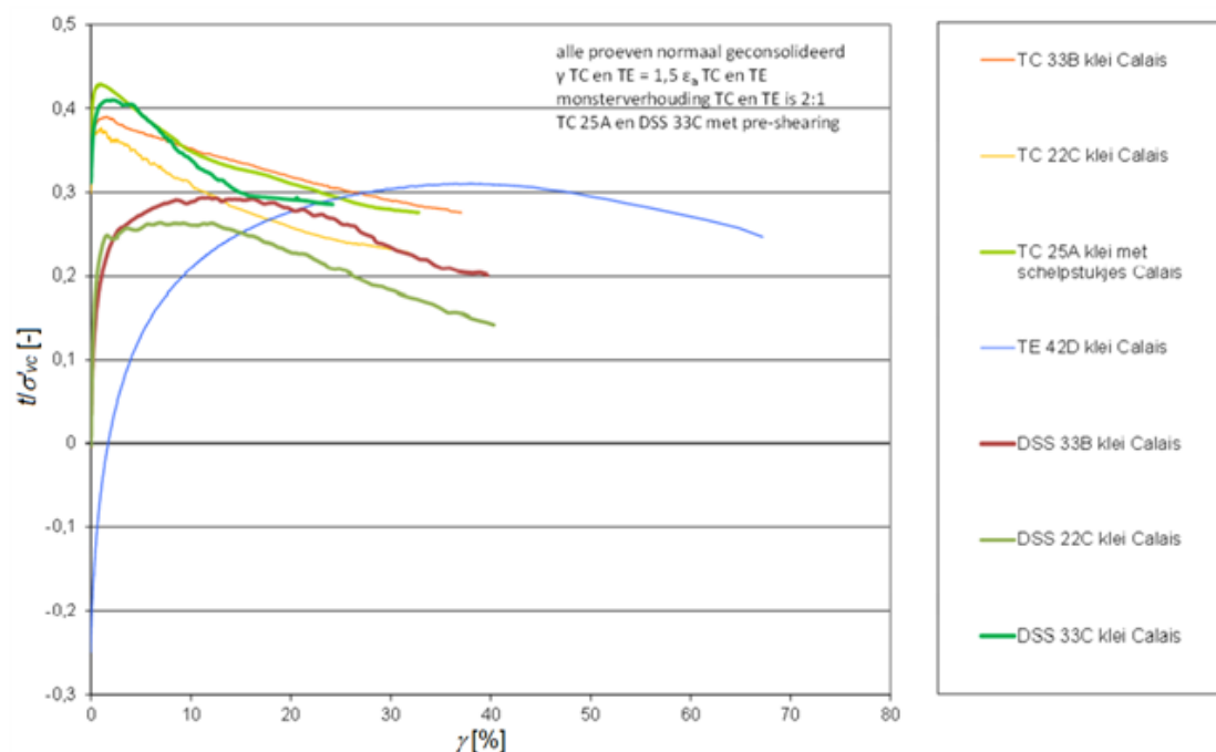
Figuur 1 Genormaliseerde schuifspanning tegen schuifrek op basis van resultaten van triaxiaal compressie proeven, direct simple shear proeven en triaxiaal extensie proeven op klei
