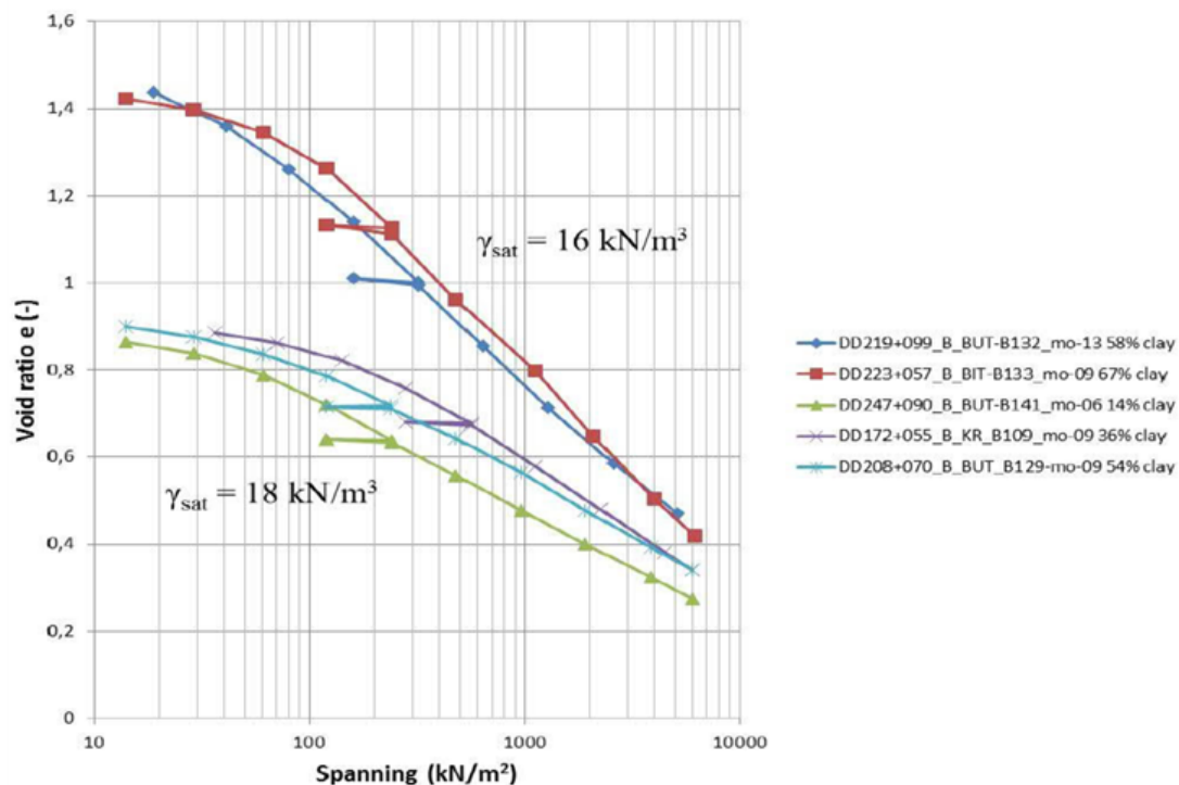
Figuur 3 Voorbeelden van samendrukkingscurves van siltige klei in het bovenrivierengebied
