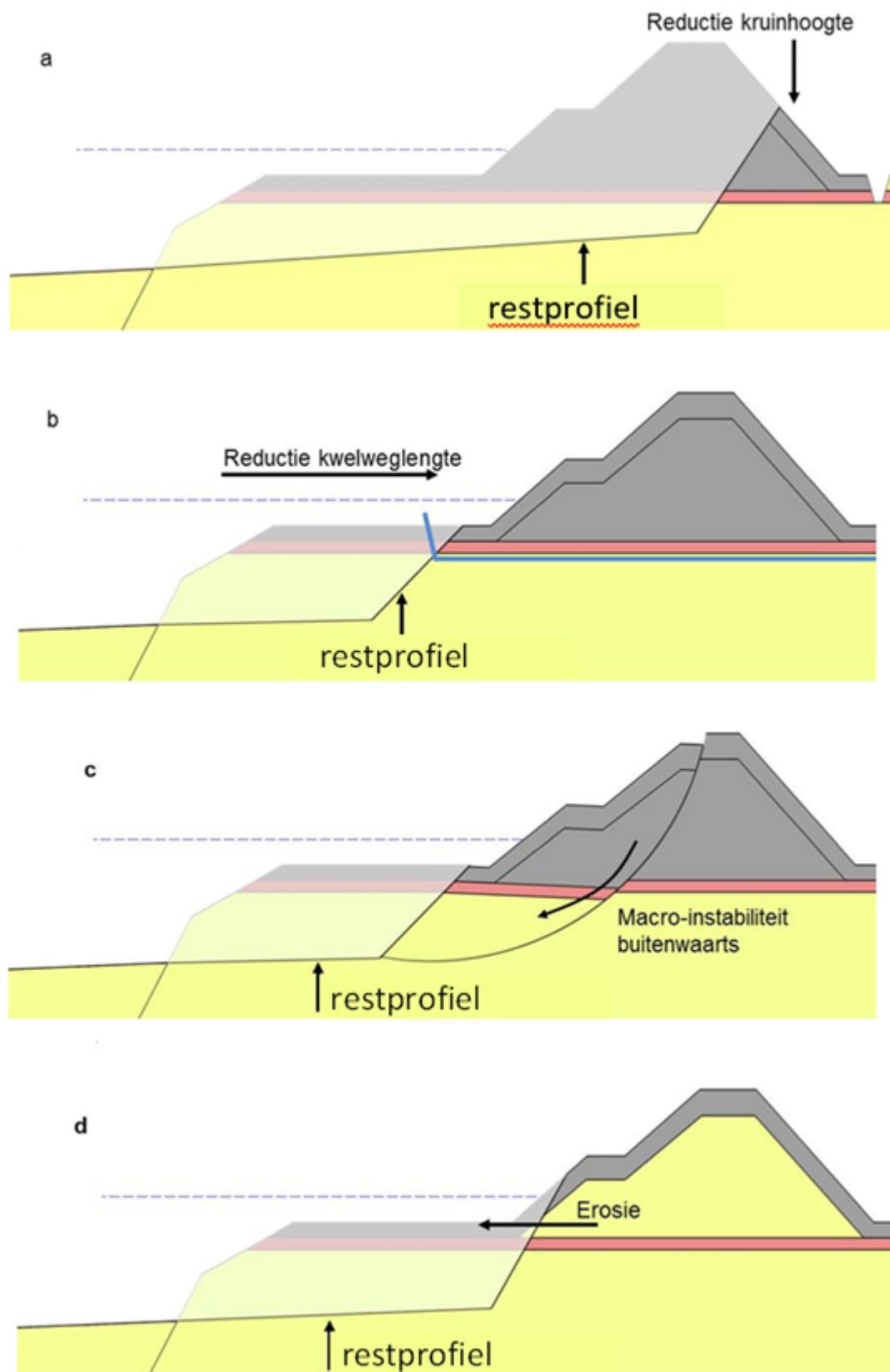
Figuur 2 Vier voorbeelden waarbij het aangetaste dijkprofiel (voorheen ook wel restprofiel genoemd) vier verschillende vervolgmechanismen beïnvloedt.
