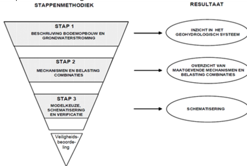
Figuur Stapsgewijze aanpak voor het schematiseren van waterspanningen.
