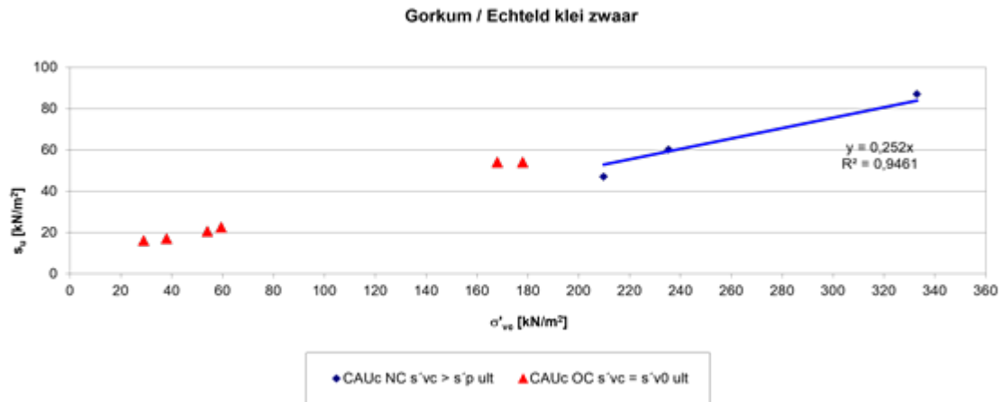
Figuur 2 Ongedraineerde schuifsterkte s_u uit de triaxiaalproeven op Gorkum klei uitgezet tegen de consolidatiespanning \sigma'_{vc} van de triaxiaalproeven; waarden bij 25% axiale rek.
