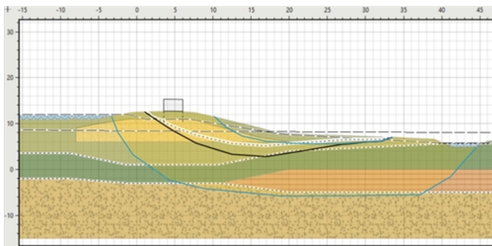
Figuur 1 Voorbeeld meest kritische afschuiving langs een vrij glijvlak.
