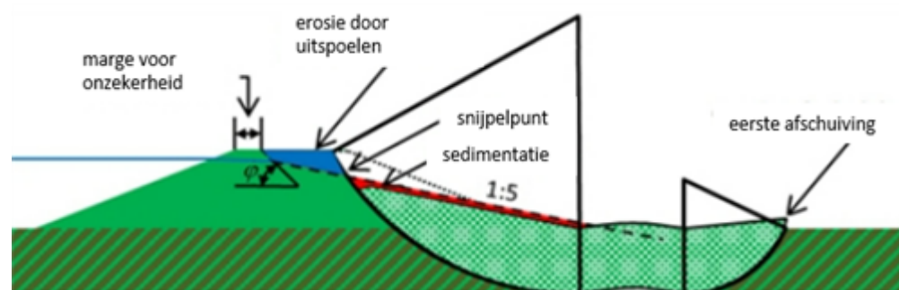
Figuur 1 Uitspoelen na afschuiving binnenwaarts.
