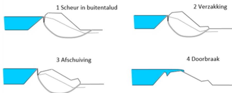
Figuur 1 Mogelijk faaltraject bij intredepunt schuifvlak in het buitentalud.
