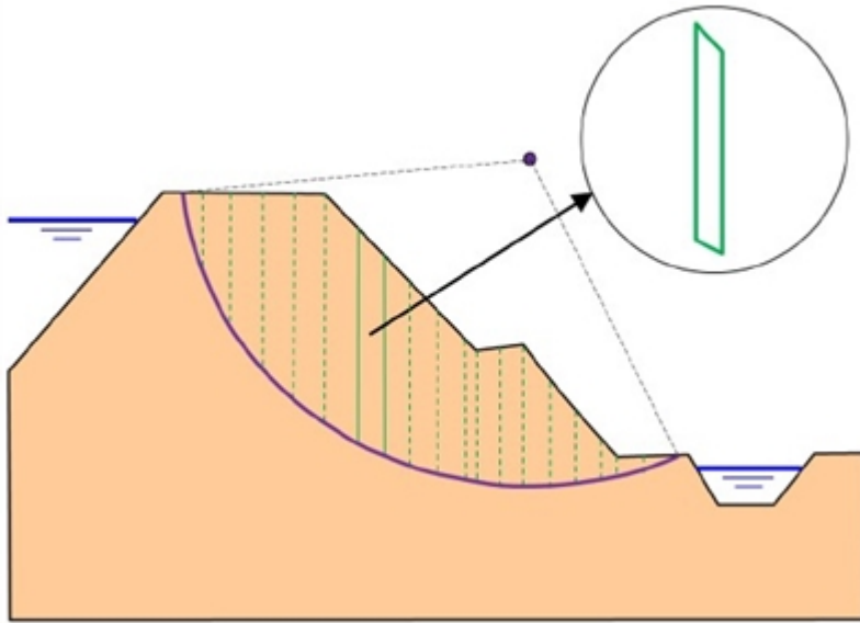
Figuur 1 Dijk met cirkelvormig schuifvlak, waarbij de afschuivende moot grond is onderverdeeld in verticale lamellen.
