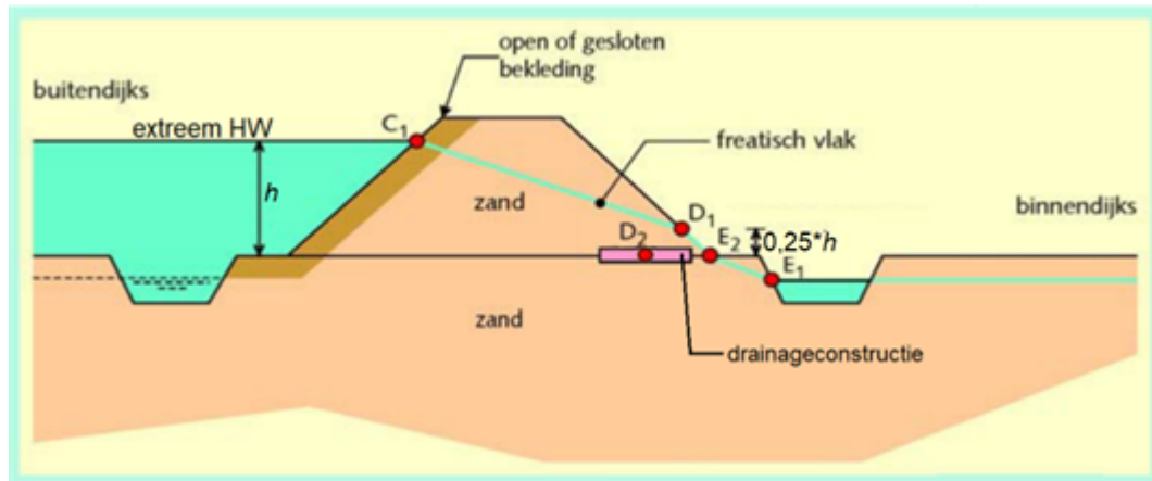
Figuur 4 Freatisch vlak voor geval 2B
