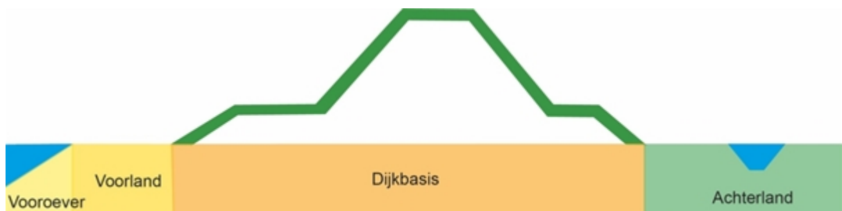
Figuur 1 Schematisatie van het dwarsprofiel.
