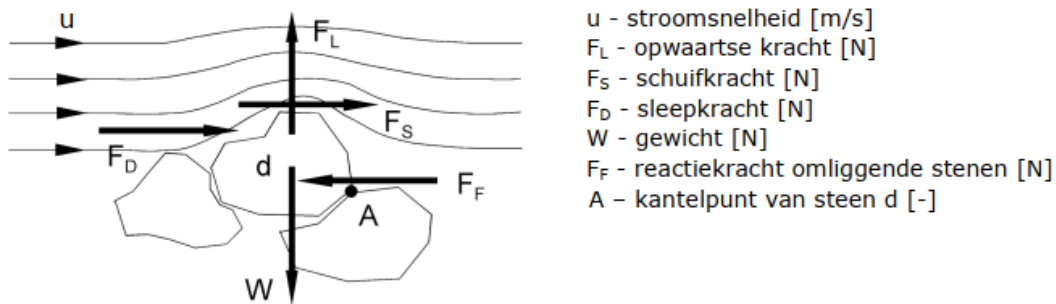
Figuur 2: Strooming en krachten voor een steen
