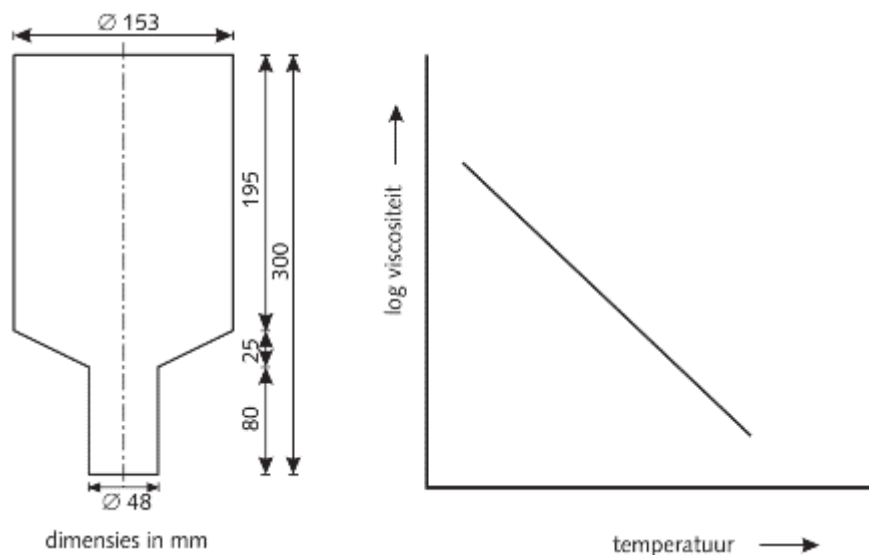
Figuur 1 Uitloopviscosimeter.
