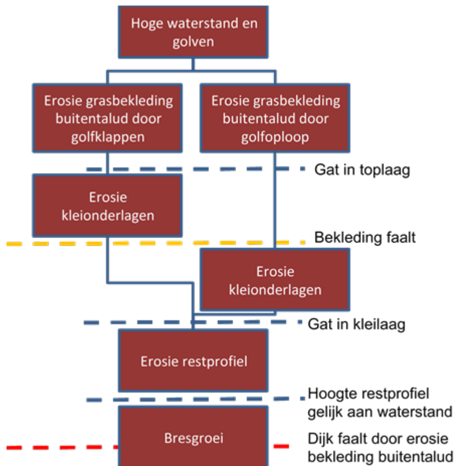
Figuur 4 Faalpad van dijk als gevolg van erosie van de grasbekleding op het buitentalud.
