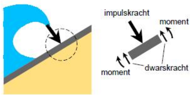
Figuur 4: Schematisering krachtenspreiding plaatbekleding
