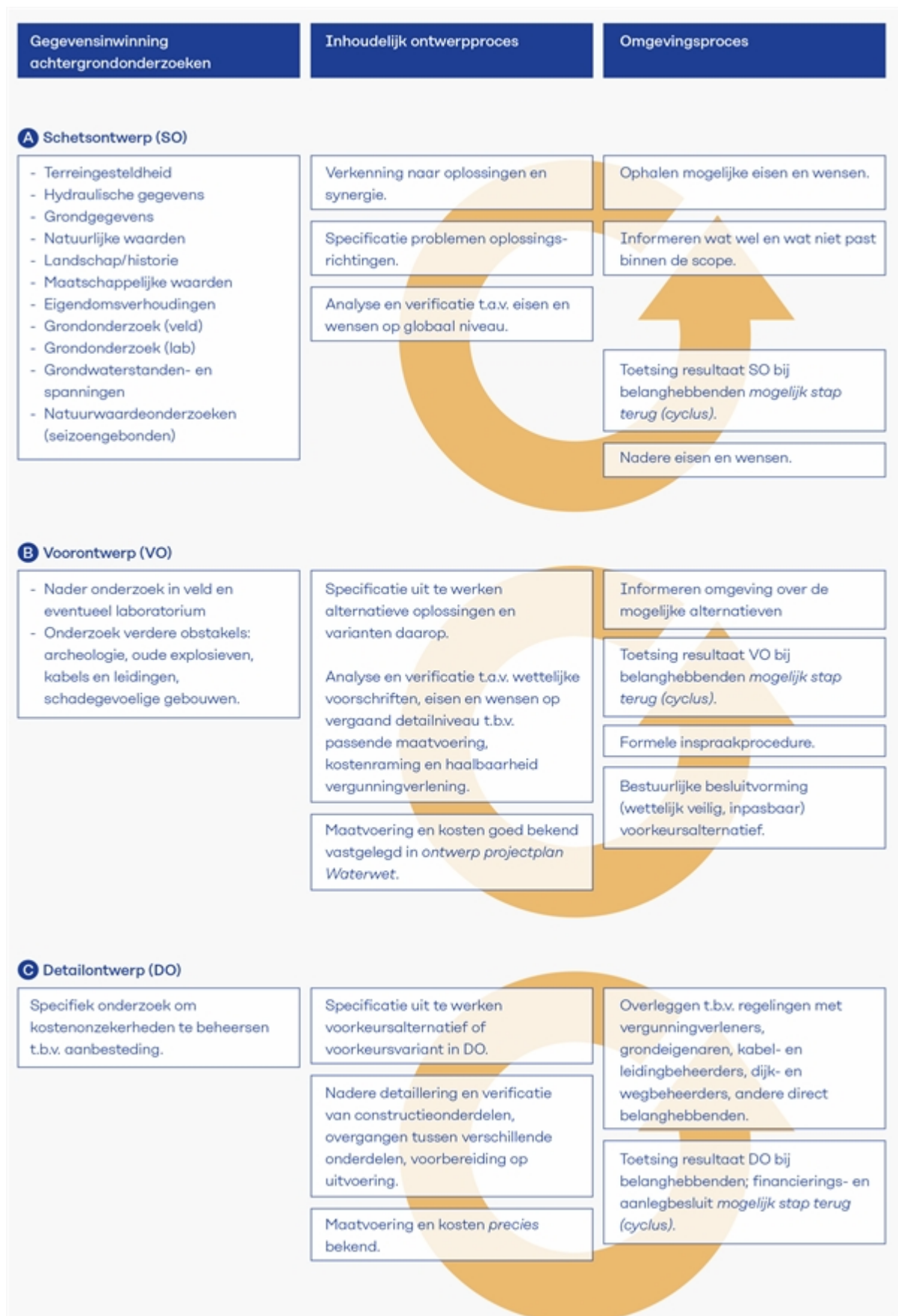
Figuur 1 Schematische weergave van het ontwerpproces.
